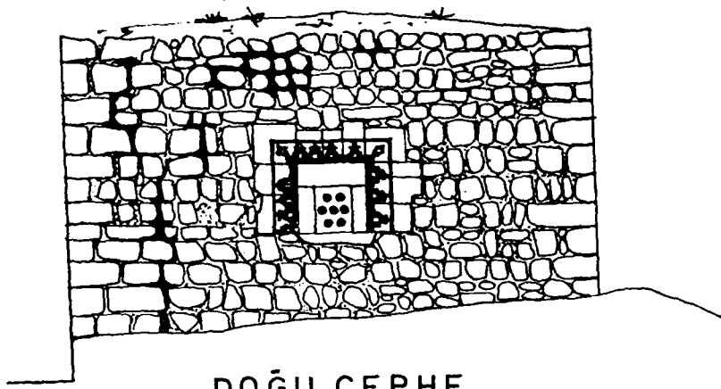
DOĞU CEPHE
