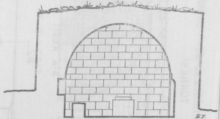
A-A KESİT
