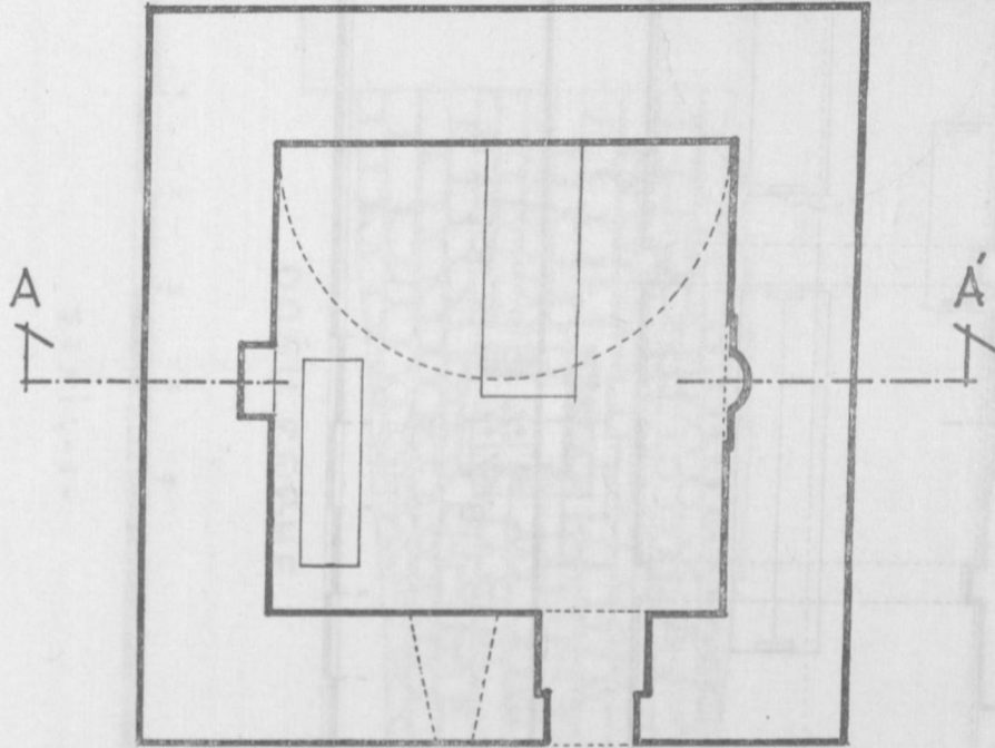
PLÂN
