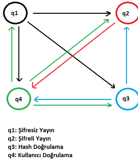
Şekil 3.6: Kılıç güvenlik ve gizlilik senaryoları arası geçiş kuralları
