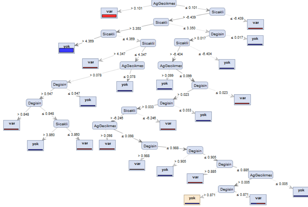
Şekil 4.8: Tekrarlama saldırısı Karar Ağacına uygulandığında oluşan ağaç
