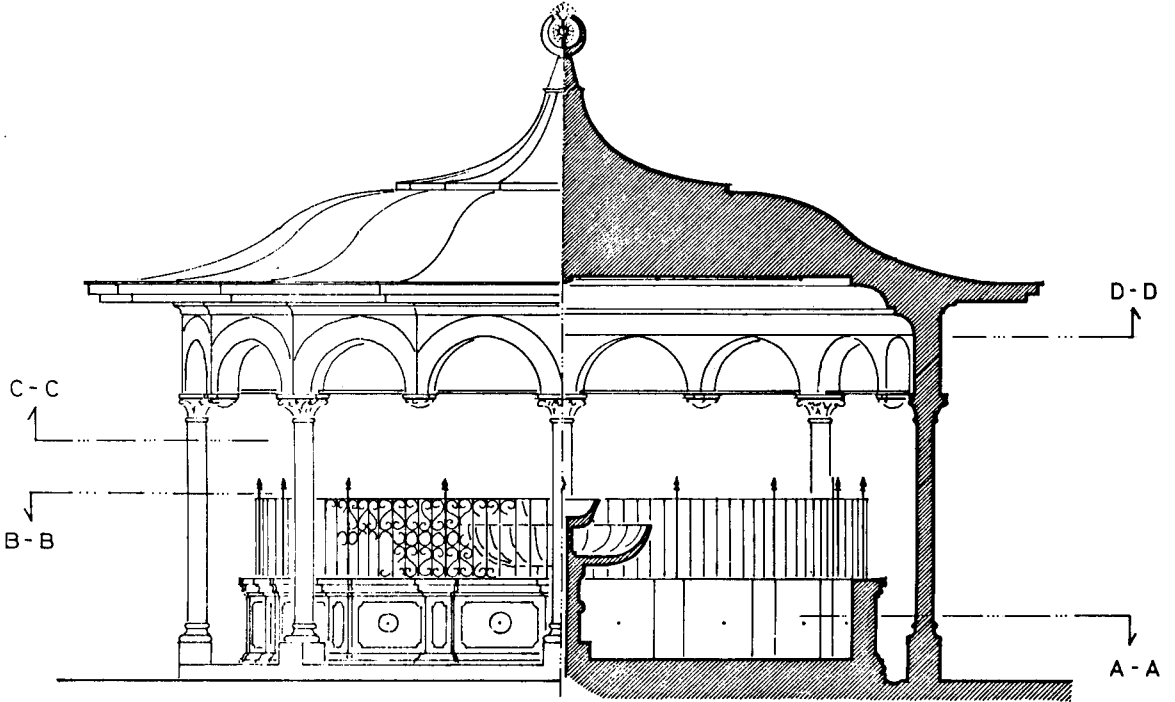
Kısmî cephe
