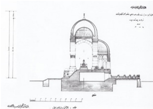
Çizim 11-12: Vakıflar Genel Müdürlüğü Türk İnşaat ve Mimarlık Eserleri Müzesi'nde Bulunan Mimar Kemalettin'in Elinden Mahmut Şevket Paşa Türbesi Plan ve Kesiti Y. YAVUZ, s. 182.
