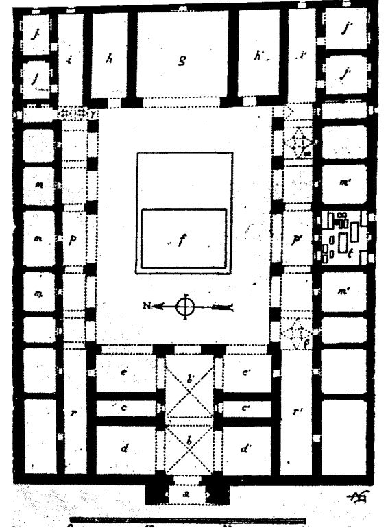
8 — Sivas Darüştifası plânı (A. Gabriel)
