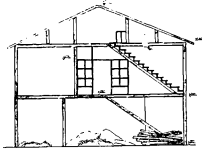
B-B KESİTİ
