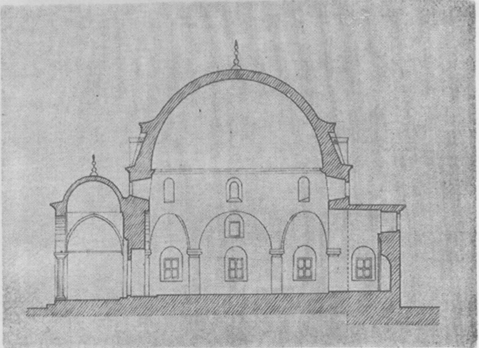
Resim : 4 — Camiin uzunlamasına kesiti.
