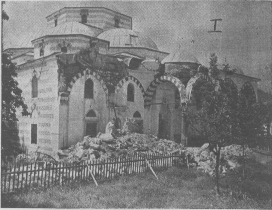
Resim : 5 — Mer'aşi Abdurrahman Paşa camii: 1943 depreminin son zana umumi görünüşü.
