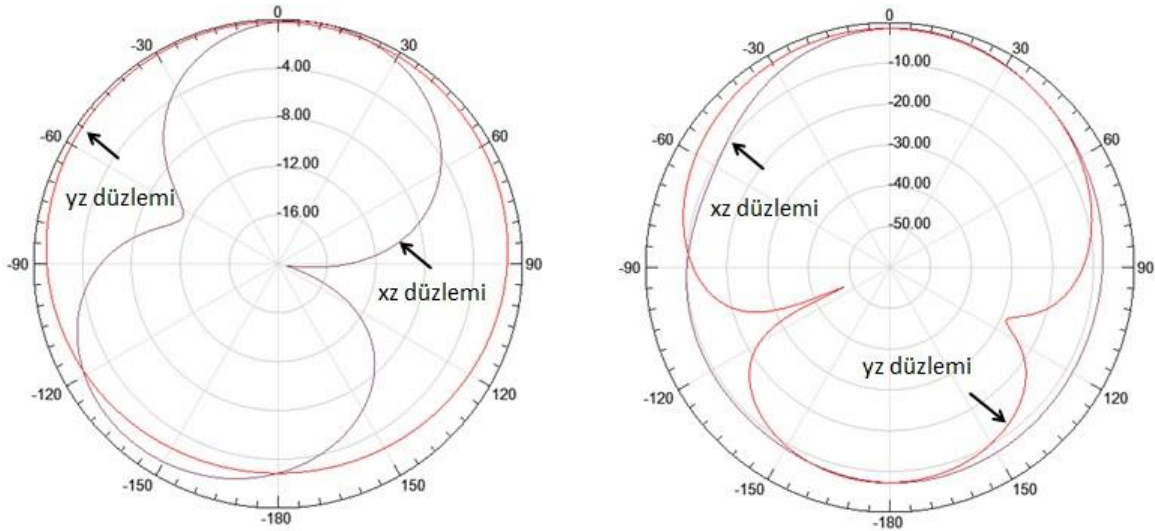
Şekil 3. (a) 403 MHz'deki ve (b) 2.45 GHz'deki xz ve yz düzlemlerindeki normalize ışınma örüntüleri
