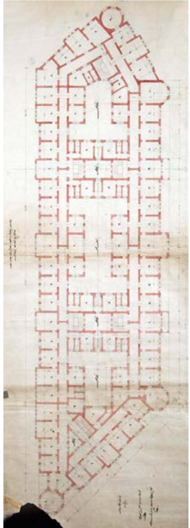
Beyoğlu Tepebaşı civarında, Sultan II.Bayezid Vakfından boş arsa üzerine yapılması tasarlanan apartman projesi (Ali Talat Bey, 1909, Vakıflar Arşivi)
