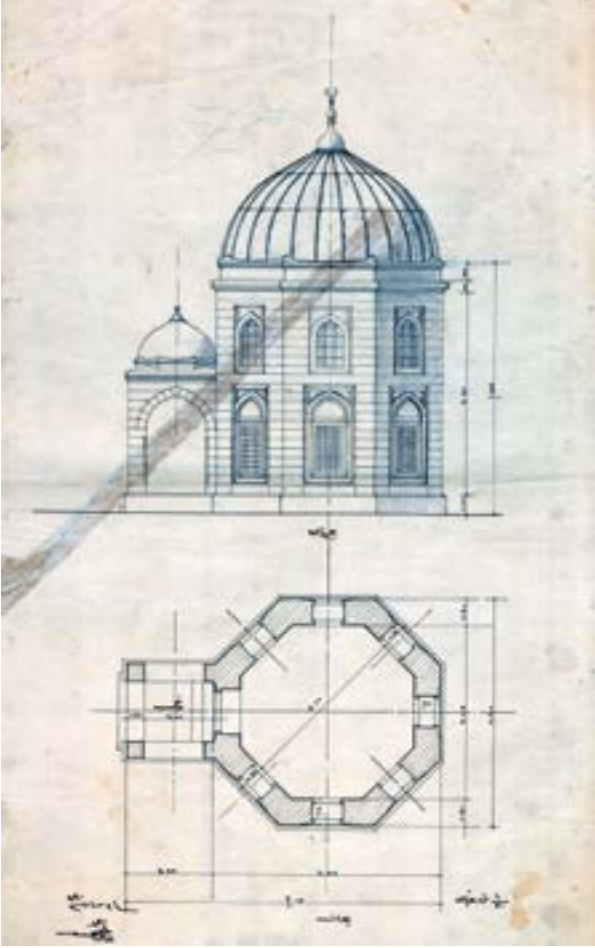
Nezaret Döneminden Barbaros Hayreddin Türbesine ait proje (Ali Talat Bey, Vakıflar Arşivi)
