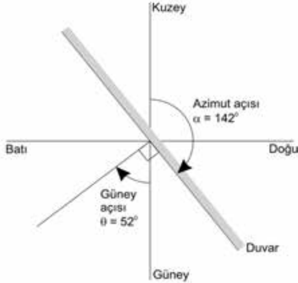
Şekil 4. Saat yüzeyinin azimut ve güney açısı.
