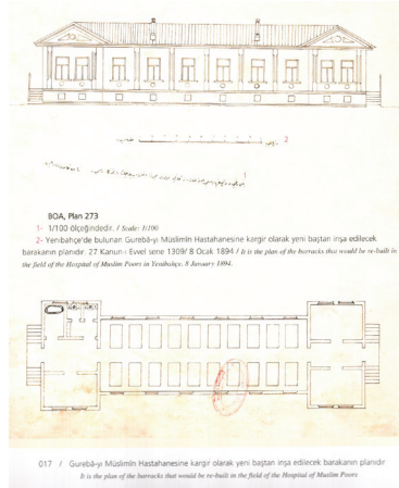
Resim 13: Bezm-i Alem Valide Sultan Hastahanesi'ne kargir olarak yeni baştan inşa edilecek barakanın cephe ve planı. (BOA. Pl.273)
