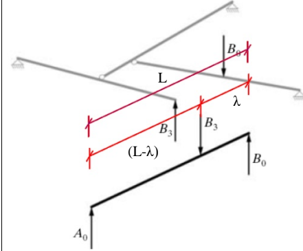
Şekil 4.22 : Bir kiriş üzerinde yük dağılımını etkileyen oranlar işaretlenmiştir[Kohlhammer, Kotnik s:83].
