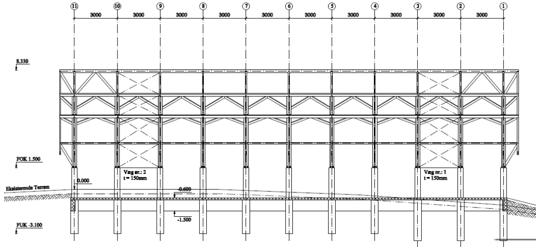
Şekil 5.3 : Mütakabil kafes kirişe dönüştürülen önerinin boy kesiti[Larsen, 2015 s:5]
