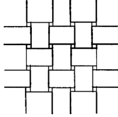
Şekil 4.42 : Sağa doğru ve sola doğru modüllerden oluşmuş bir mütakabil yapıdır [Baverel ve diğ, s:157]
