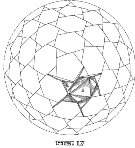
Şekil 3.12 : 270 çubuktan üretilen jeodezik kubbenin plan görünüşü [ABD Patenti No:3063521]
