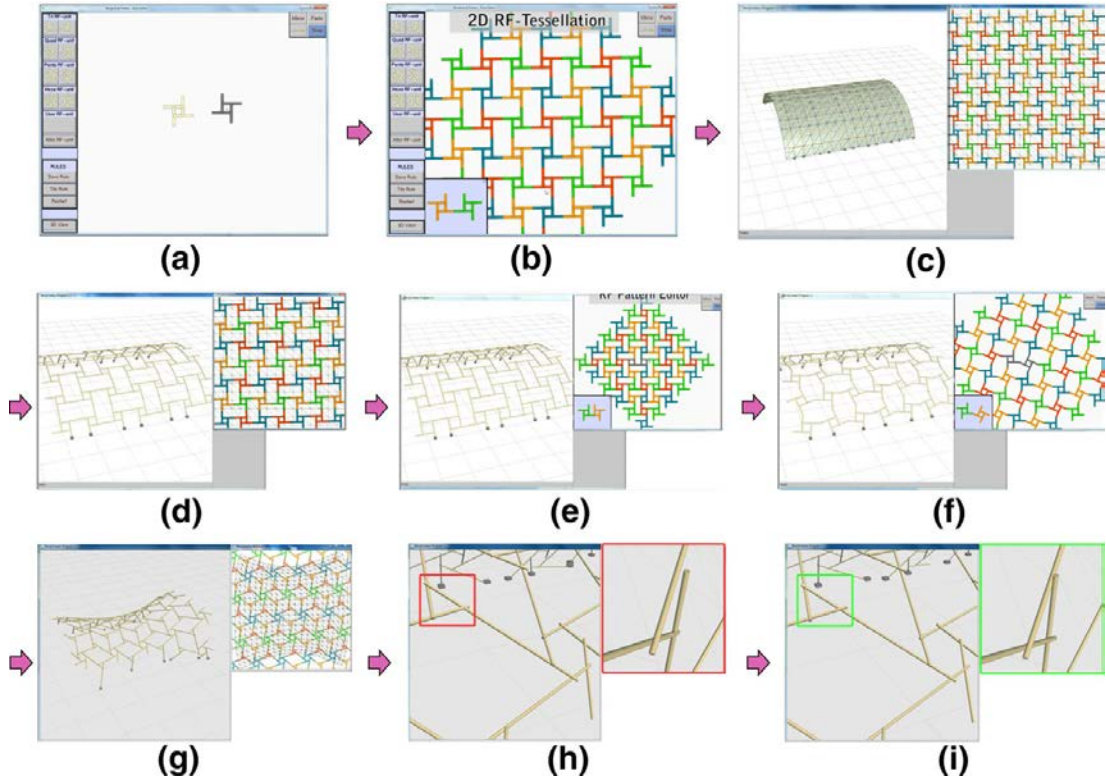
Şekil 3.35 : a–c arası mütakabil sisteme uygun bir mozaiklemenin üretilmesi ve tahmini bir üç boyutlu kılavuz yüzeyin üzerine haritalanması, d–f çeşitli parametrelerin interaktif biçimde değiştirilmesiyle tasarımın görünüşü üzerinde rötuş yapılması; g–i optimizasyon aracı uygulanarak aynı düzlemde ve bağlantılı çubuklar elde edilmesi. [Song ve diğ. s:115]
