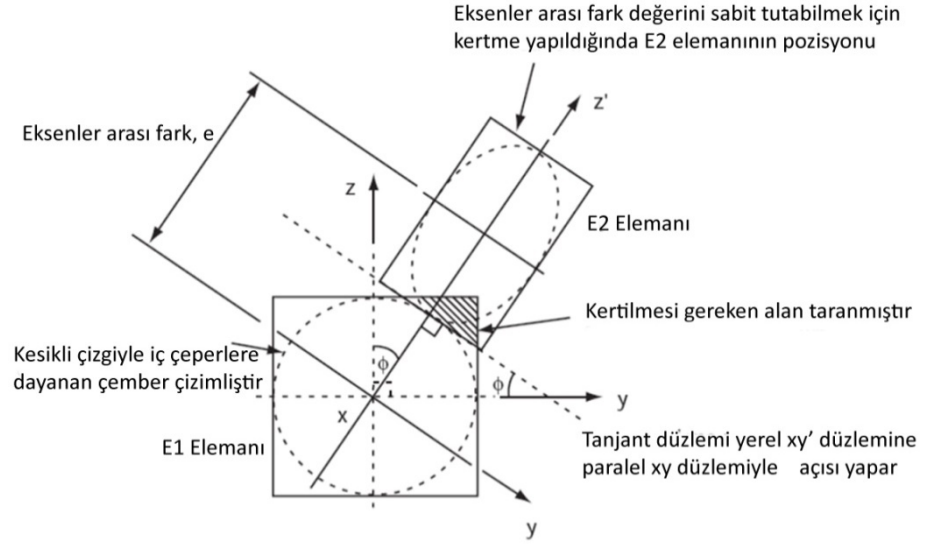
Şekil 4.57 : Çok merkezli bir mütakabil strüktürün bağlantı noktasından alınan kesitte kertilmesi gereken alan taranmıştır[Rizzuto, Larsen s:251]
