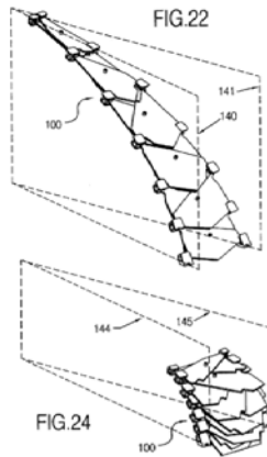
Şekil 3.51 : Yarım ve tam açık kısıpçaıla bağılı eğimli bir dilimi gösteren perspektif görünüşü [ABD Pantenti No:6739098]
