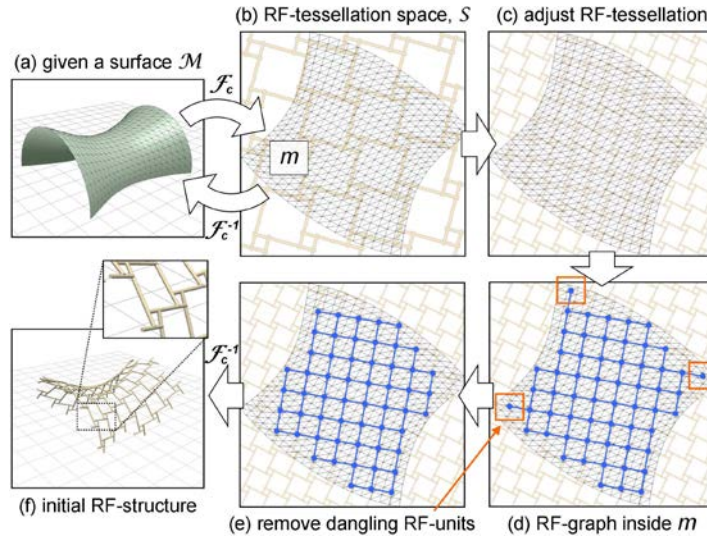
Şekil 4.30 : Bir hiperboloidin haritalanması[Song ve diğ. s:5]
