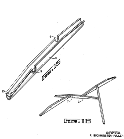
Şekil 3.1 : Gerilim bütünlüğü kompleksini oluşturan birbirine bağlı kollarin (Görsel no. 15) bir araya gelişi perspektif görünüm (Görsel no. 16) [ABD Pantenti No:3063521]
