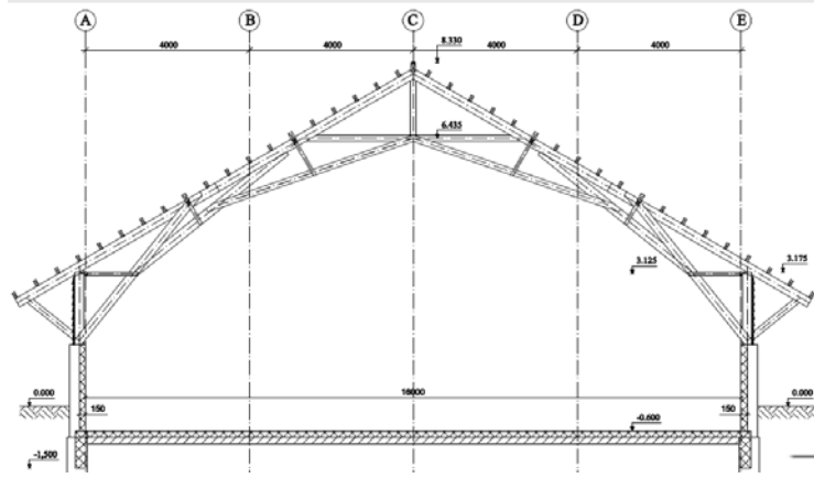
Şekil 5.2 : Mütakabil kafes kirişe dönüştürülen önerinin enine kesiti[Larsen, 2015 s:5]
