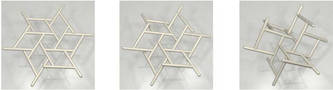
Şekil 4.82 : İki boyutlu kirişlemenin üç boyutlu strüktüre dönüşümü [Roelofs, 2008 s:23]
