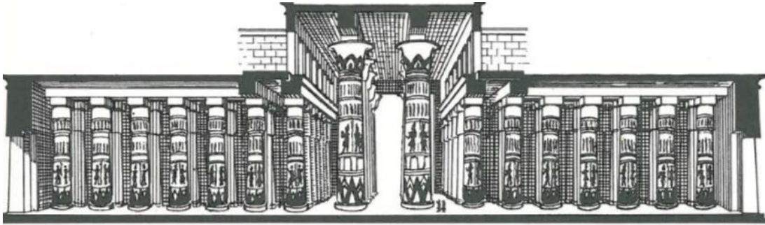
Şekil 2.10 : Karnak, Amon tapınağının hipostil salonun kesiti, M.Ö.1312-1301 [Lloyd, s:31]
