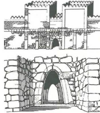
Şekil 2.9 : Boğazköy, tapınağın kral kapısı. Kulelerle desteklenen eliptik açıklık, bindirme kemer ve yekpare taş söveden oluşur[Lloyd s:26].
