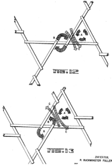
Şekil 3.11 : Gerilim bütünlüğü kollarının bitişlerinde basıncın oluşturduğu dönme eğilimini gösteren diyagramlar [ABD Patenti No:3063521]
