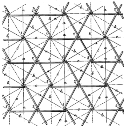
Şekil 3.38 : Açık strüktürün kısmi plan görünüşü [ABD Pantenti No:3185164]
