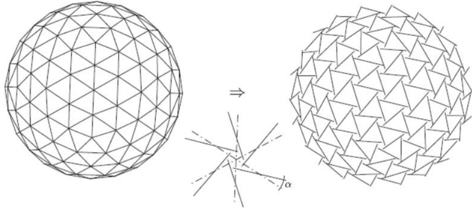
Şekil 3.28 : Bir jeodezik kürenin yarısından, kenarların döndürülmesi yöntemiyle ( \alpha:\pi/10 açısı kadar döndürülmesiyle) elde edilen mütekabil kubbe strüktür [Brocato, Mondardini s:1788]
