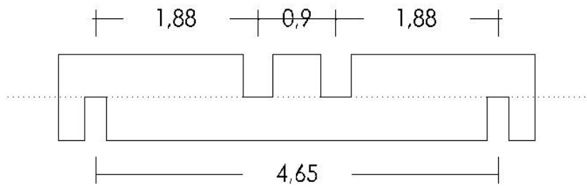
Şekil 4.73 : Maket çalışması için seçilen kiriş boyutları incelendiğinde kiriş boyunun (L) 4.65cm; bağlantı mesafesinin ( \lambda ) 1.88cm; eksenler arası fark (e) değerinin 0 (sıfır) olduğu görülür.
