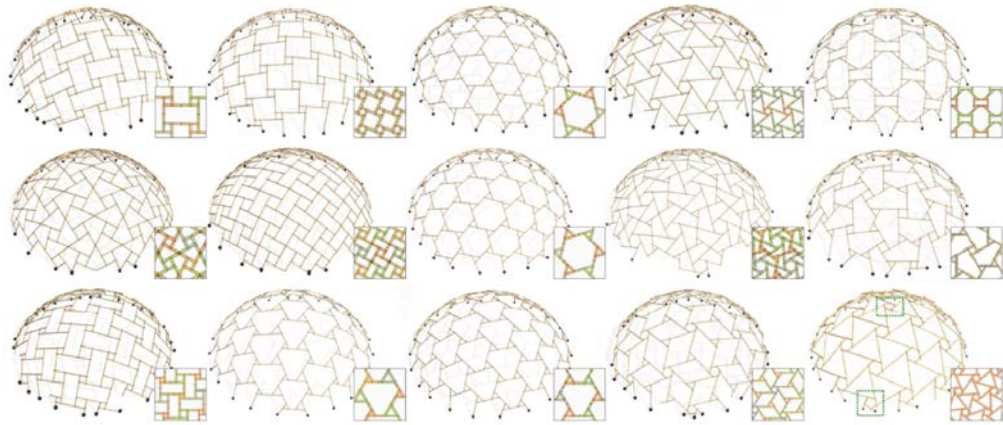
Şekil 4.31 : Bir kubbenin çeşitli kırışleme kurgularına uygun olarak haritalanması[Song ve diğ. s:8]
