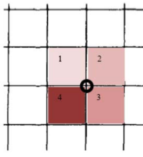
Şekil 4.67 : İşaretli köşede ve tüm köşelerde 4 adet kare birleşmektedir. Dizilim; 4.4.4.4 veya 4^4 şeklinde kodlanır [Grünbaum, Shephard s:229]
