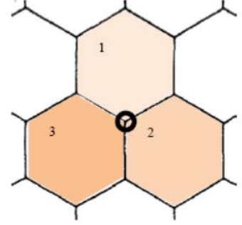
Şekil 4.68 : İşaretli köşede ve tüm köşelerde 3 adet altıgen birleşmektedir. Dizilim; 6.6.6 veya 6^3 şeklinde kodlanır [Grünbaum, Shephard s:229]
