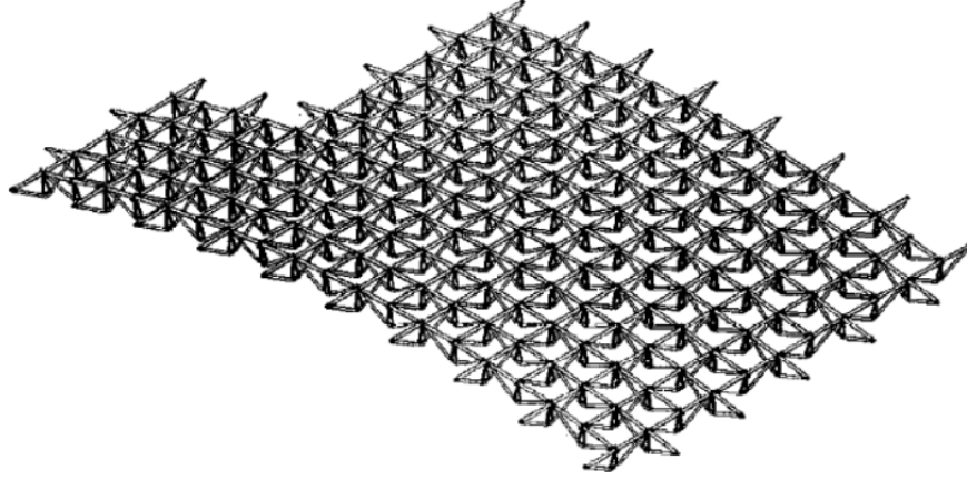
Şekil 4.25 : Mütəkabil çatı strüktürünün perspektif çizimi [Gelez, Aubry ve Vaudeville s:306]
