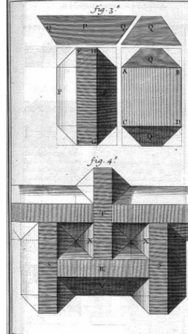
Şekil 2.27 : Strüktürü oluşturan taşların görünüşü[Fleury s:2]
