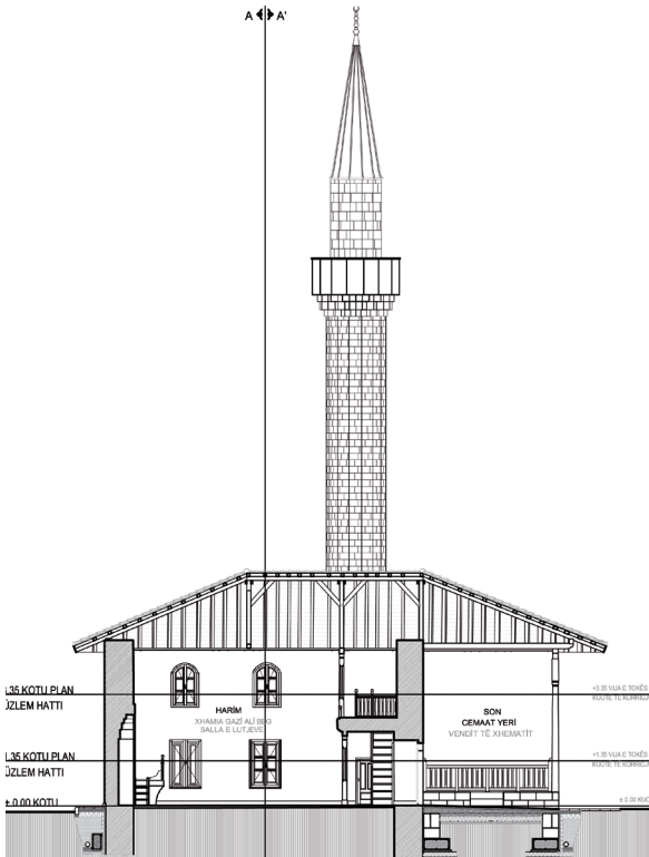
Şekil 18. Gazi Ali Bey Cami restorasyon projesi, BB kesiti (AY-MİR Mimarlık Müh. Ltd. 2015).
