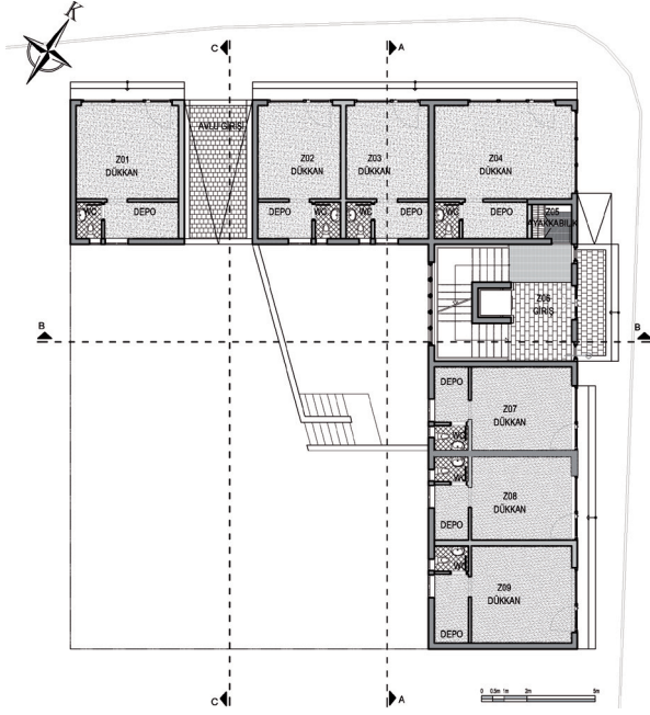
Şekil 22. Gazi Ali Bey Camisi ek binaları, Viçitırın İslam Topluluğu Binası, zemin kat planı (AY-MİR Mimarlık Müh. Ltd. 2015).
