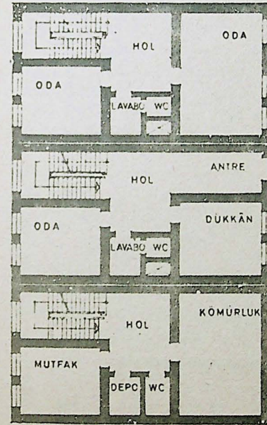
Akaretlerde konut tipleri (İrfan, H.Bayhan., Mesken tipleri., s.31-33)
