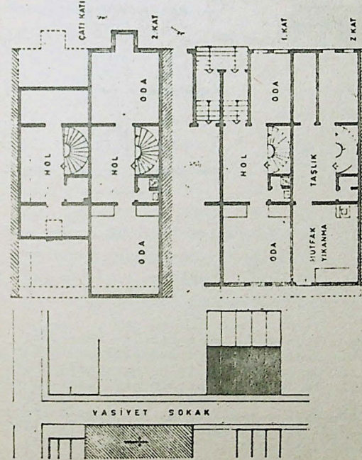
Surp-Garabet ermeni kilisesine ait konut-tipi (İrfan H.Bayhan., Mesken Tipleri..., s.164).
