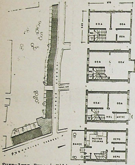
Surp-Agop Ermeni Kilisesi Vakıflarında konut tipi (İrfan H. Bayhan., Mesken tipleri., s.167).
