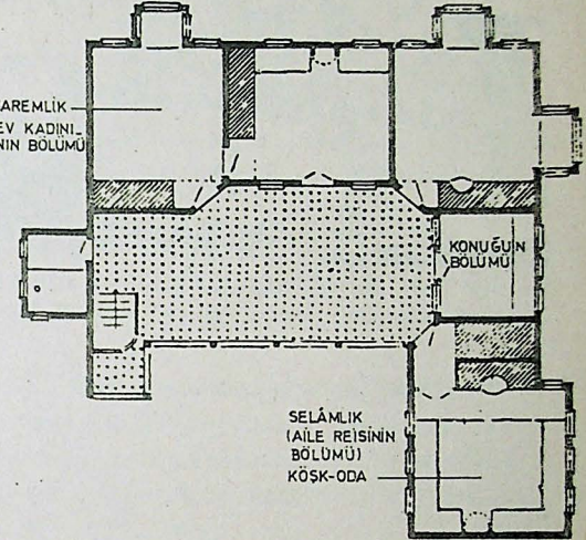
Bergama'da Hacı İsmail Ağa Konağı (Eldem, Sedat H., Türk Evi Plan Tipleri, s.60).
