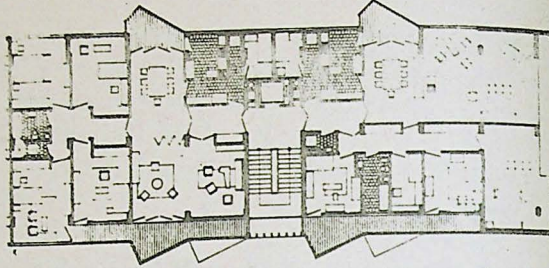
Ataköy yerleşmesi F tipi konut (Unal, Mete., İstanbul'da Apartmanın..., s. 201).
