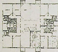
Ataköy yerleşmesi P ve S tipi konutlar (Arkitekt 1975/2, s.53-56).
