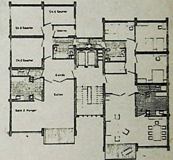
Ataköy yerleşmesi A tipi konut (Ünal, Mete., İstanbul'da Apartmanın..., s.201).
