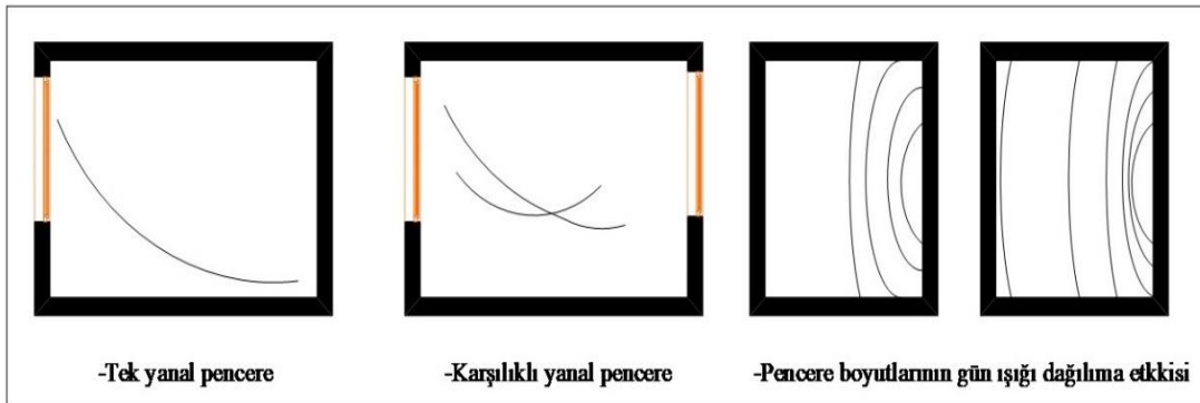
Şekil 4.2: Pencerelele plan ve kesitte günışığı dağılımları (Yener, Köknel, 2007).
