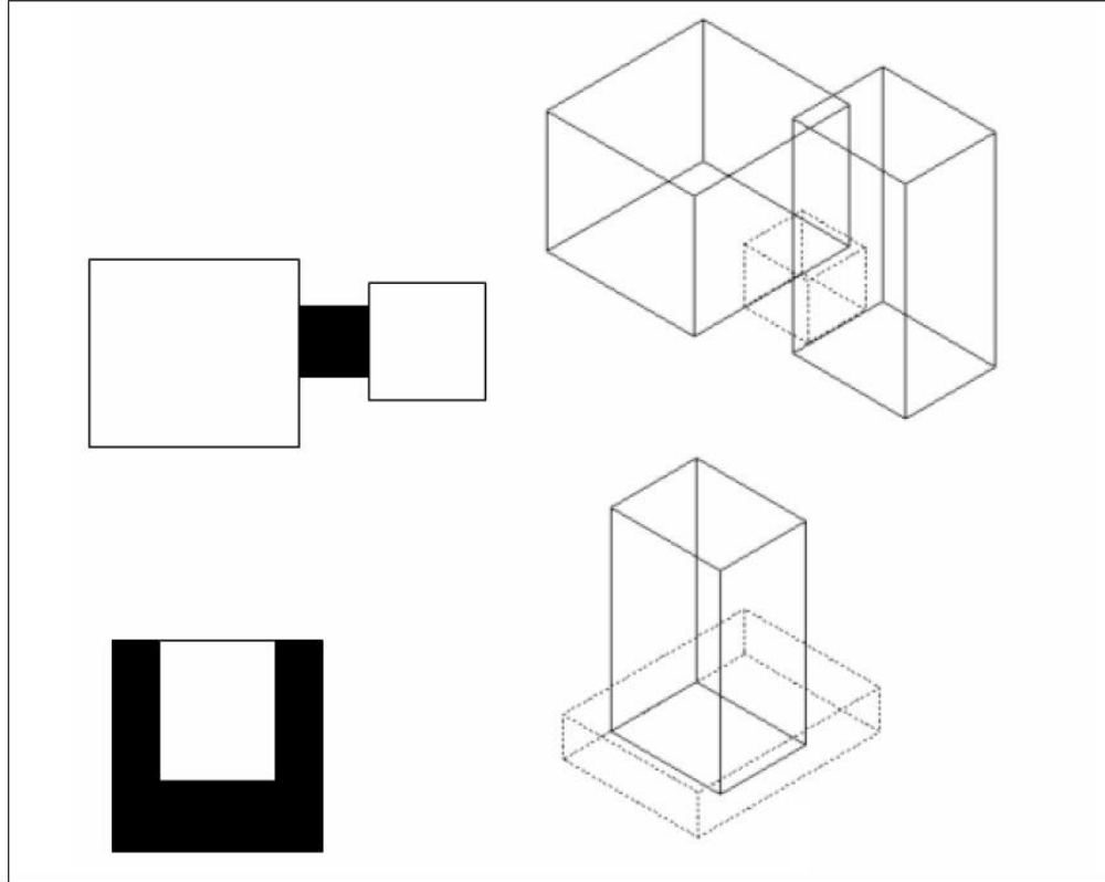
Şekil 4.10: Plaza Tipi atrium şematik planı ve perspektifi (Göçer, 2006).
