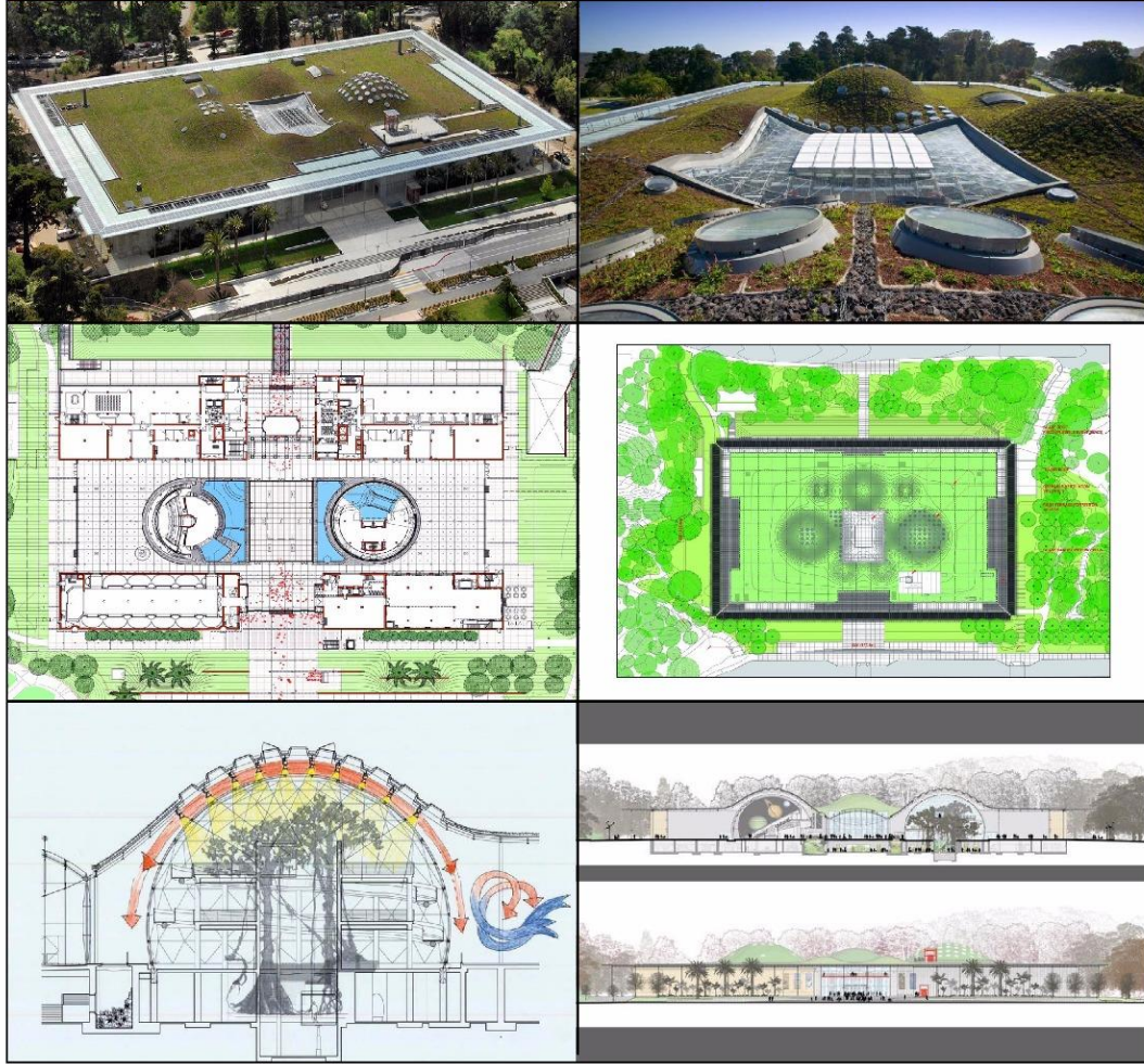
Resim 5.5: Californiya bilim akademisi ekolojik özellikleri.
