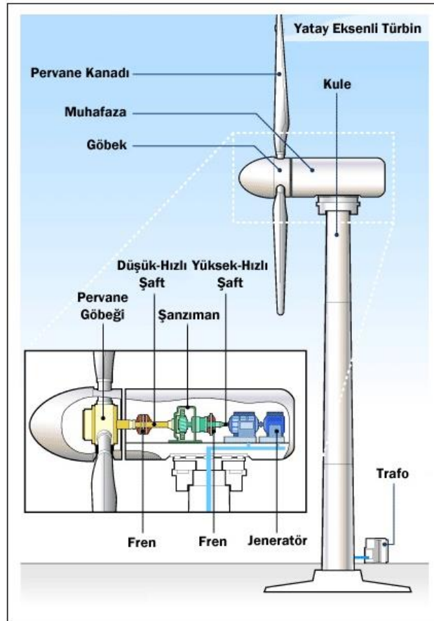
řekil 2.7: Rüzgâr türbünü (Url-2).
