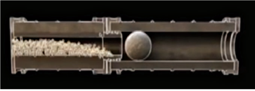
Şahi Topu Kesiti: Bakır-%10 Kalay alaşımı kovan ve namlu, mermer gülle, barut yığını.
