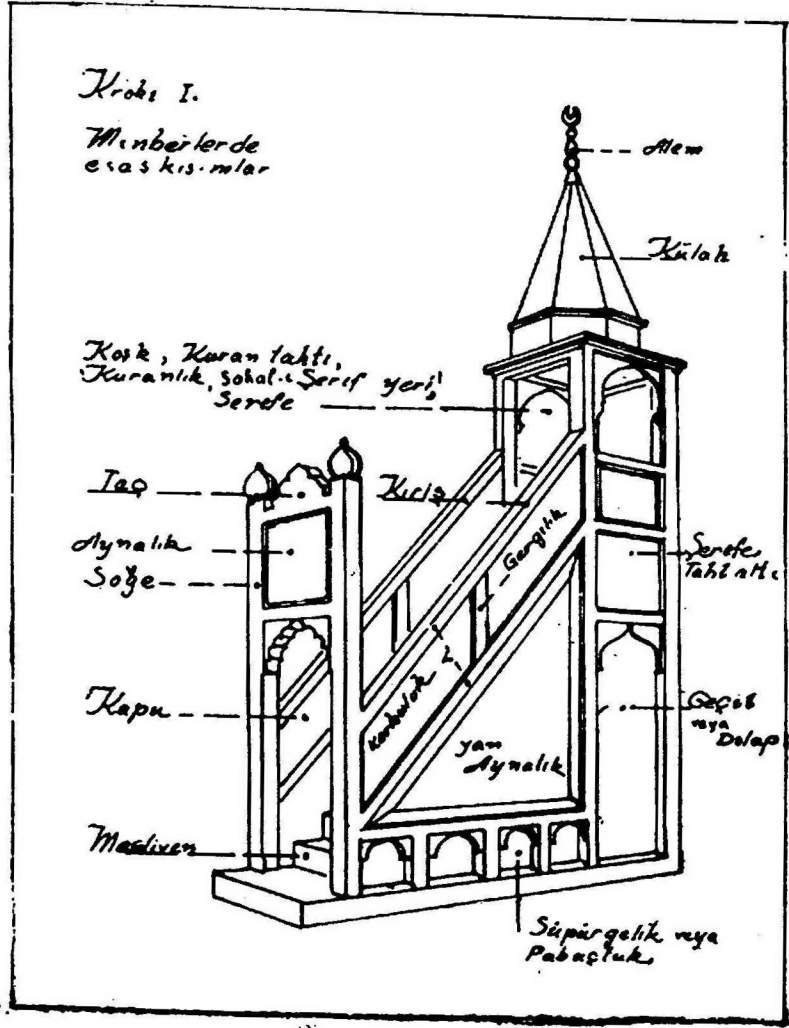
Kroki : 1 — Minberlerde esas kısımlar.
