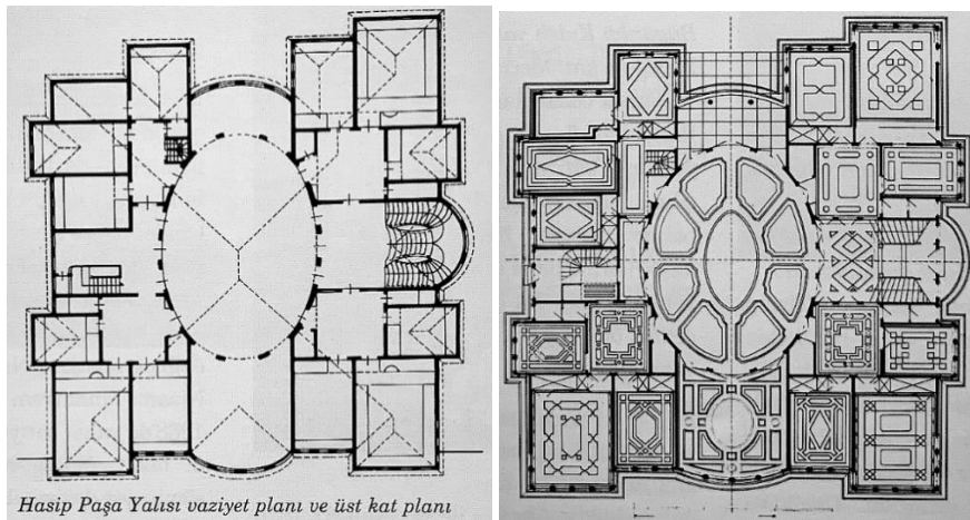
Şekil 95. Hasip Paşa Yalısı planı ve rekonstrüksiyon planı, S.H. Eldem Türk Evi (Erdenen,2006, s.298).
