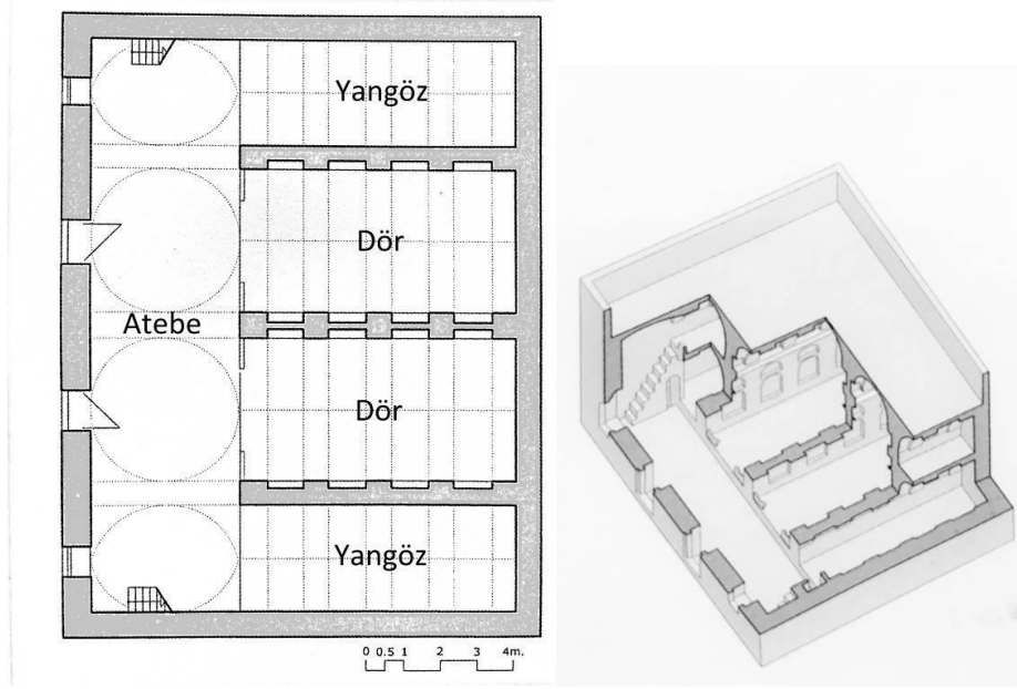
Şekil 4.6 Dört gözlü büyükev plan tipi (Saatçi, 2007)
