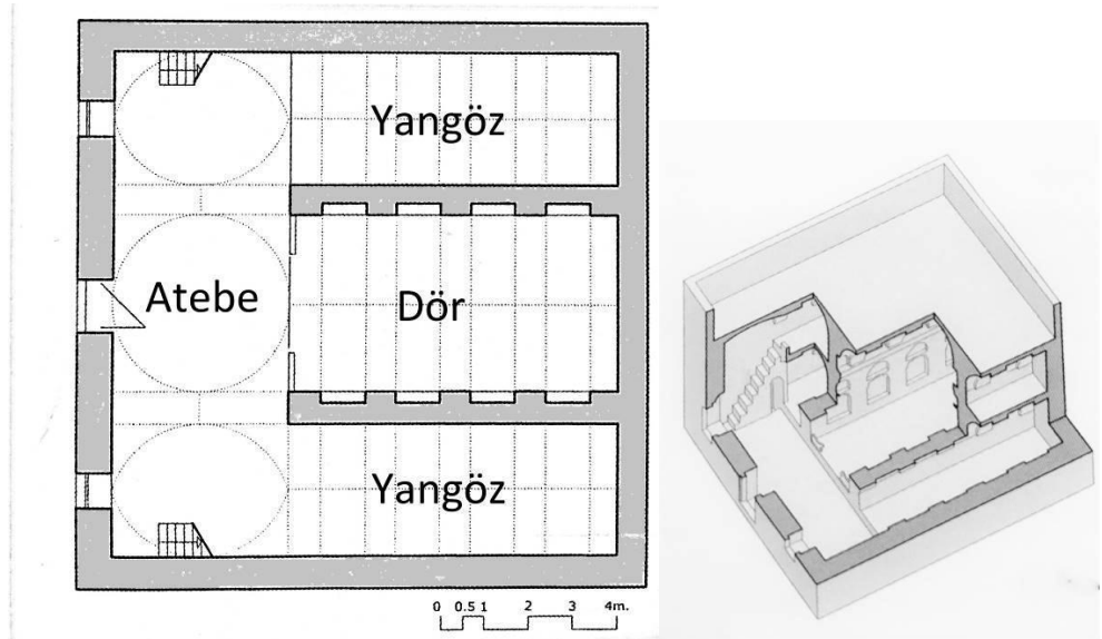
Şekil 4.5 Üç gözlü büyükev plan tipi (Saatçi, 2007)
