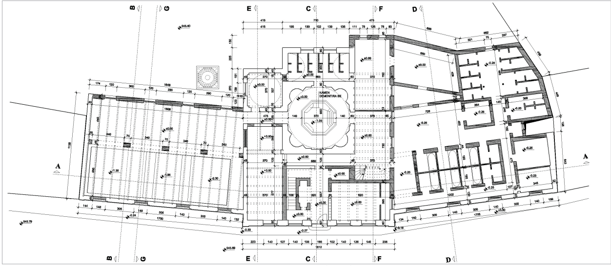
Çizim 1-Hamamın plan rölövesi.
