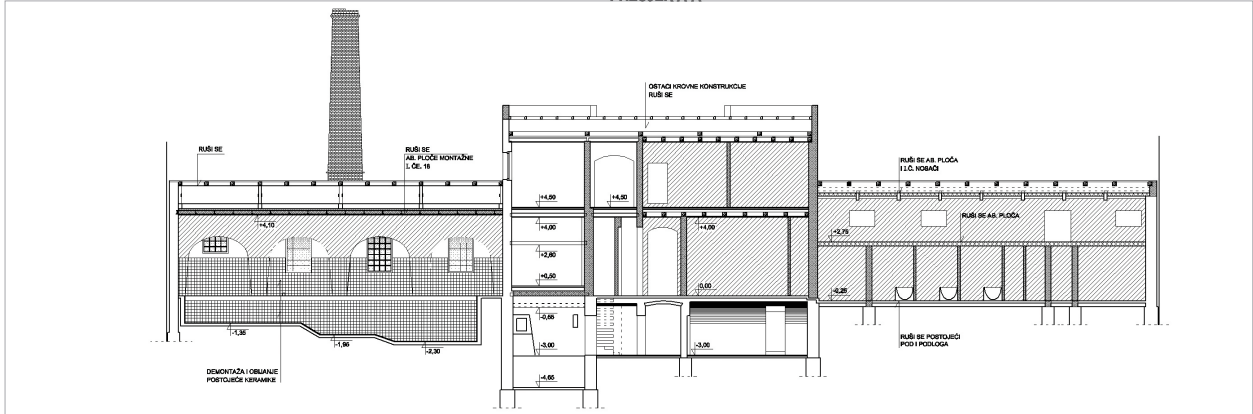
Çizim 2- Kesit rölöveleri.
