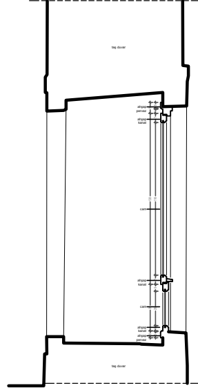
CAMİ PENCERE KESİT
