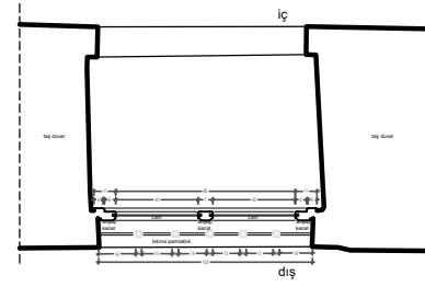
CAMİ PENCERE LOKMA PARMAKLIK PLAN
