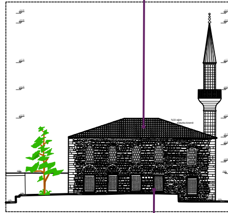
C. ÇATI ALATURKA KİREMIT OLARAK DEĞİŞTİRİLMİŞTİR VE AHŞAP ÇATI DETAYI ÇİZİLMİŞTİR.
