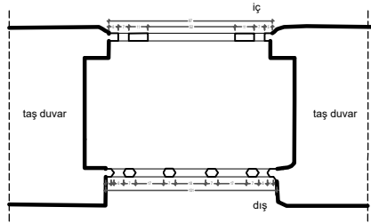
CAMİ ÜST KOT PENCERE PLAN
