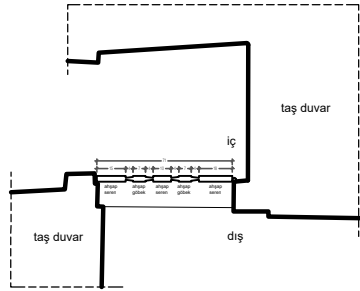
MİNARE KAPI PLAN
