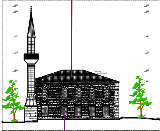
C. ÇATI ALATURKA KİREMIT OLARAK DEĞİŞTİRİLMİŞTİR VE AHŞAP ÇATI DETAYI ÇİZİLMİŞTİR.
