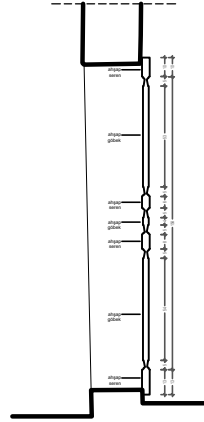
KAFE DİŐ KAPI KESİT
