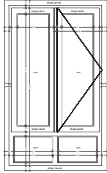
CAMİ PENCERE GÖRÜNÜŞ
