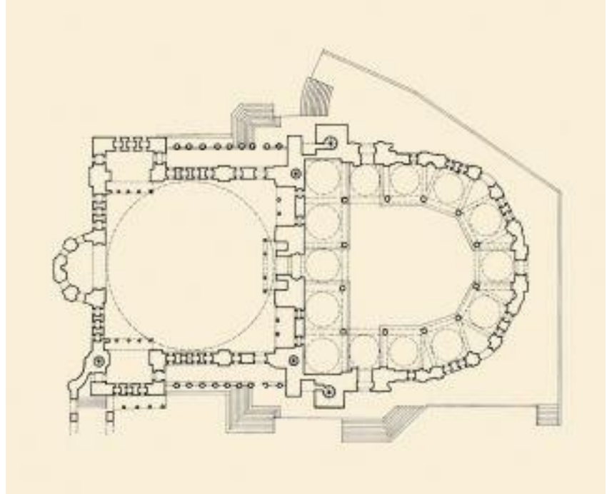
Şekil 2.2 Nuruosmaniye Cami Planı
