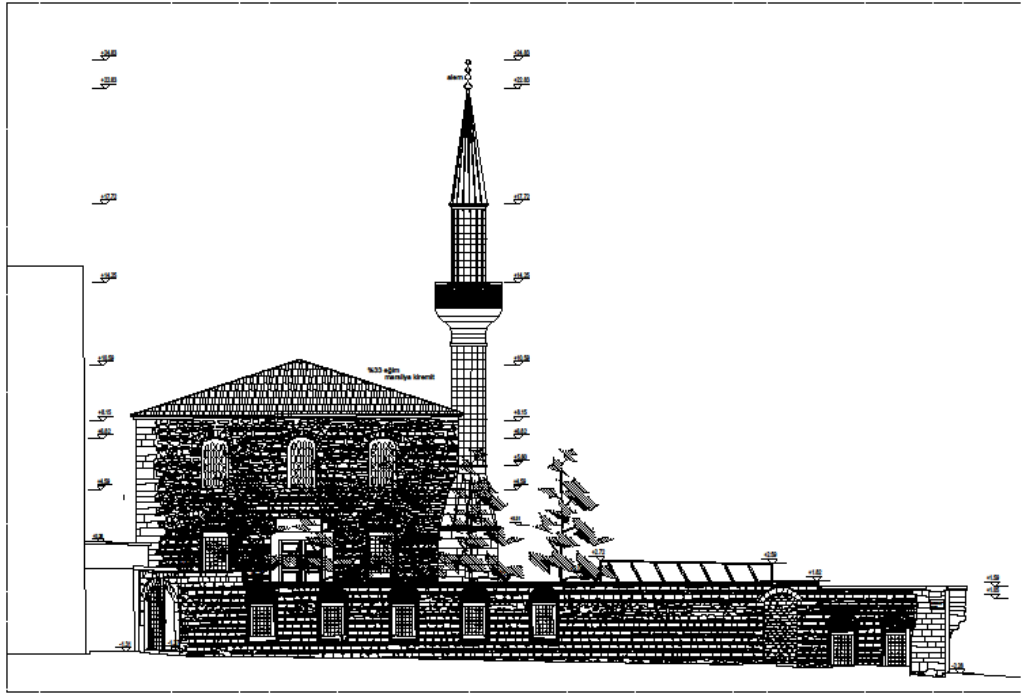
Şekil 3.54 Rölöve, Kaptanı Derya İbrahim Paşa Sokak Silüeti
