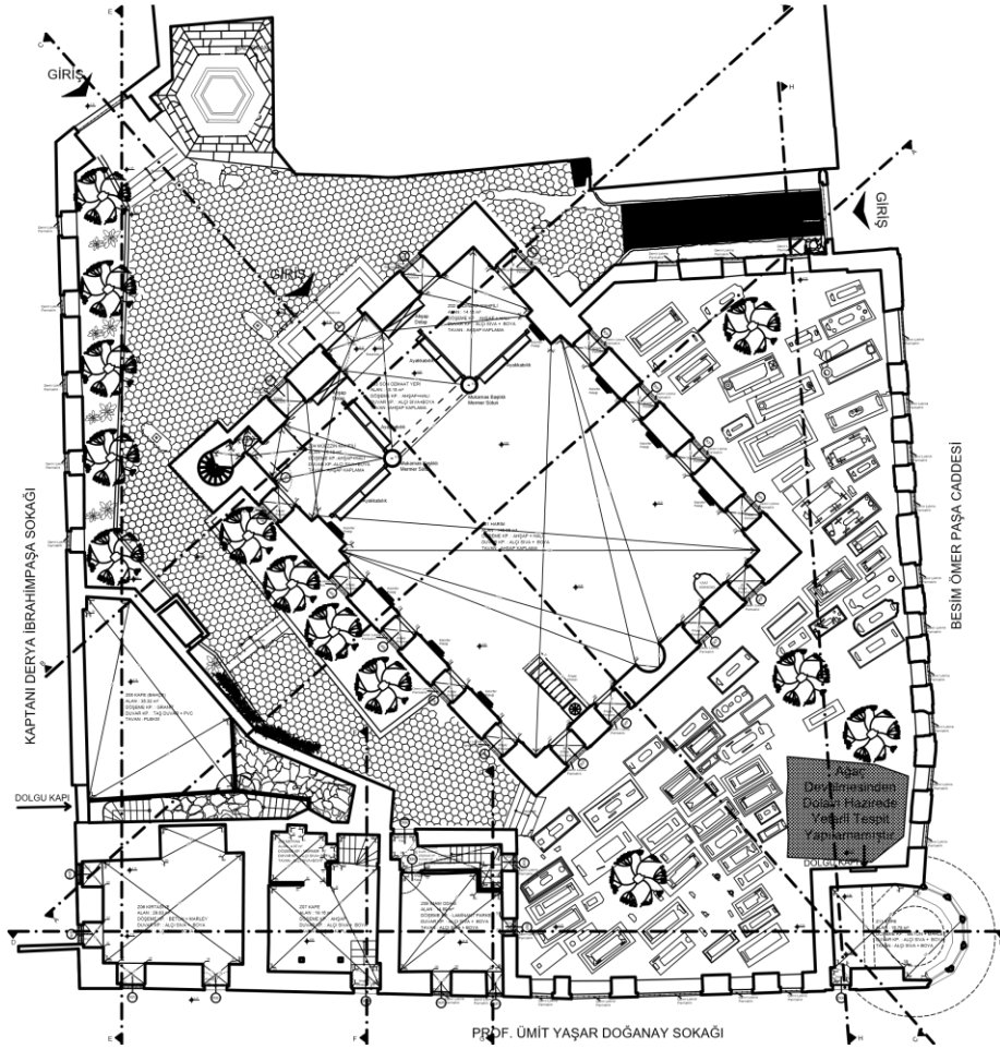
Şekil 3.12 Rölöve, Zemin Kat Planı
