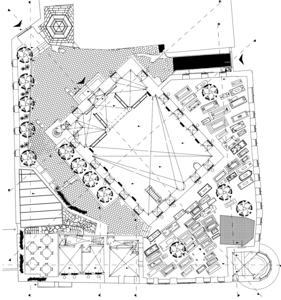
Şekil 3.38 Rölöve, Birinci Kat Planı
