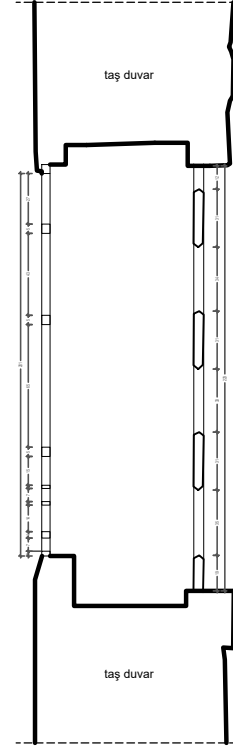
CAMİ ÜST KOT PENCERE KESİT
