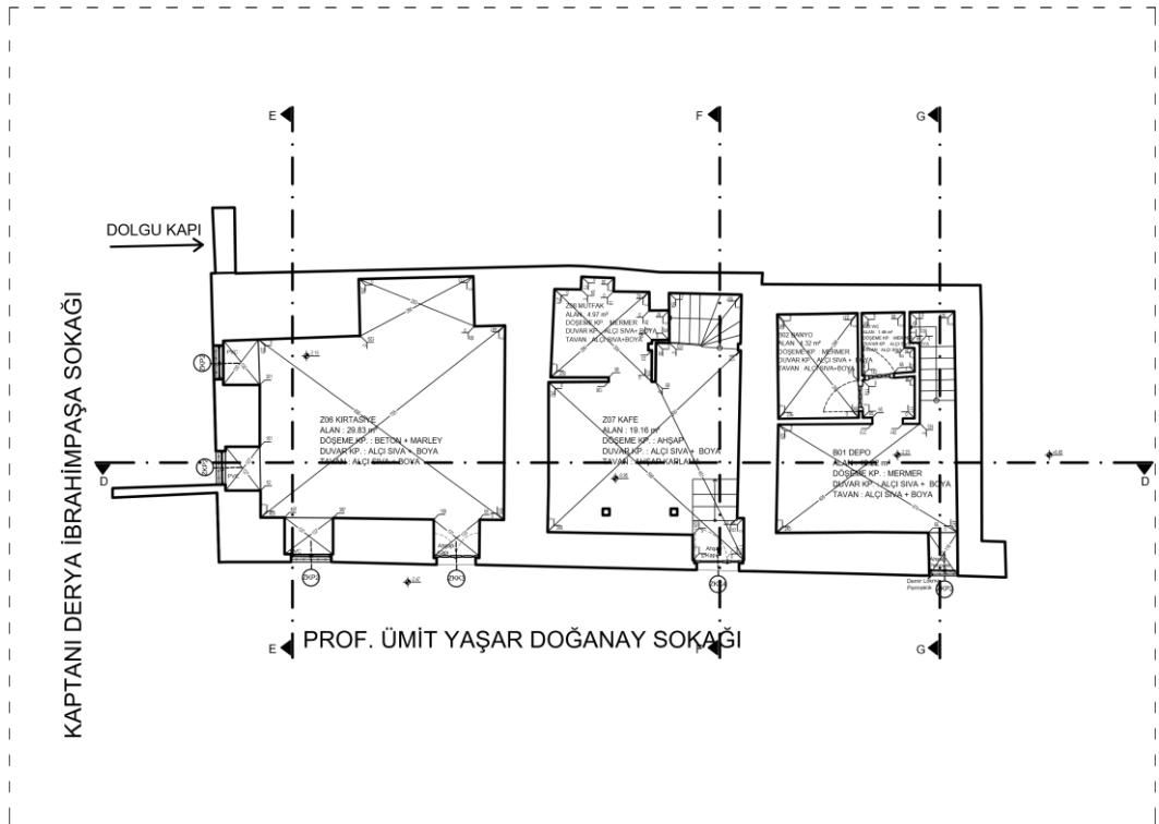
Şekil 3.7 Rölöve, Bodrum Kat Planı
