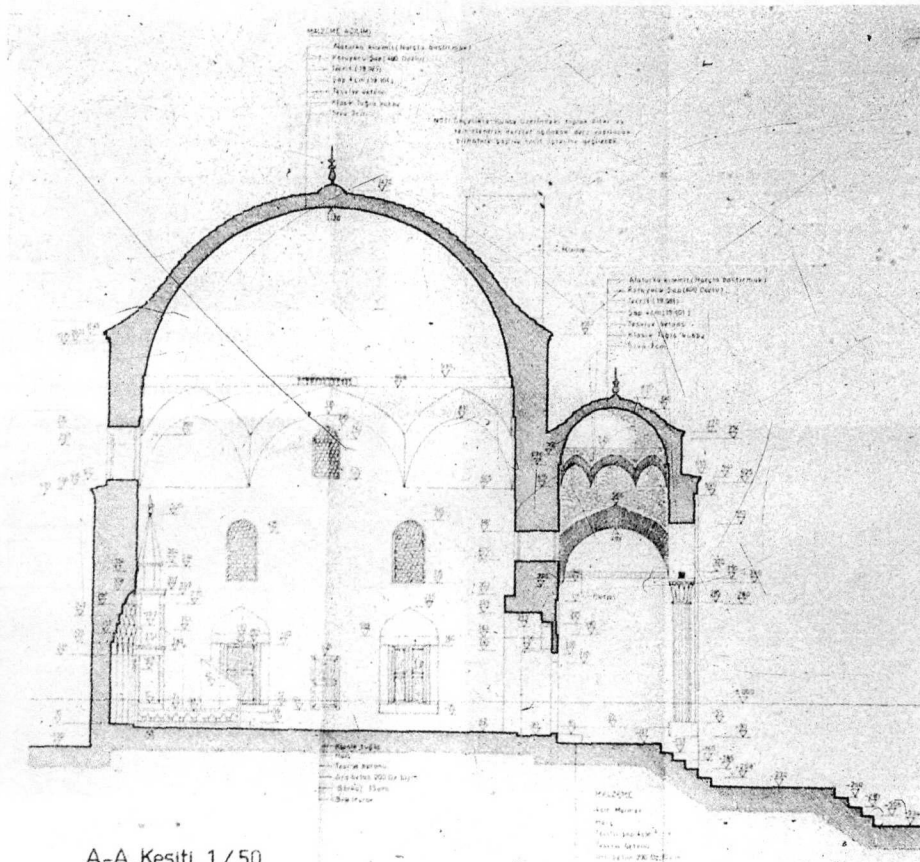
Şekil 3. Caminin kesiti.
