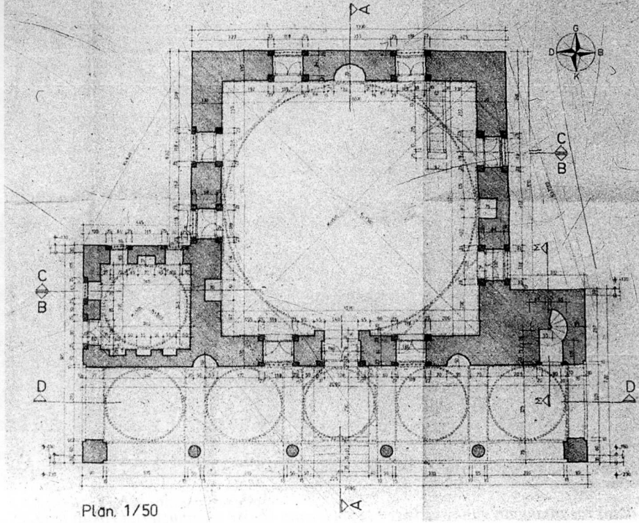
Şekil 2. Caminin planı.
