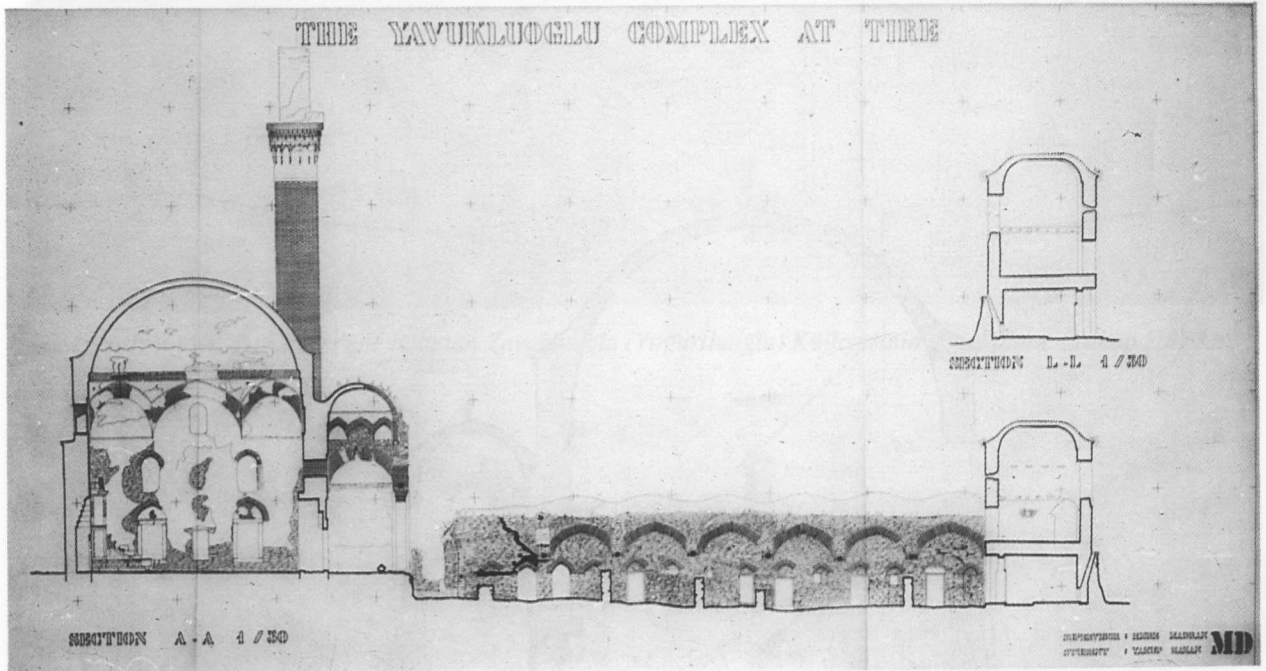
Şekil 5. Rasathanenin rölöve kesitleri. (Yakup HAZAN)
