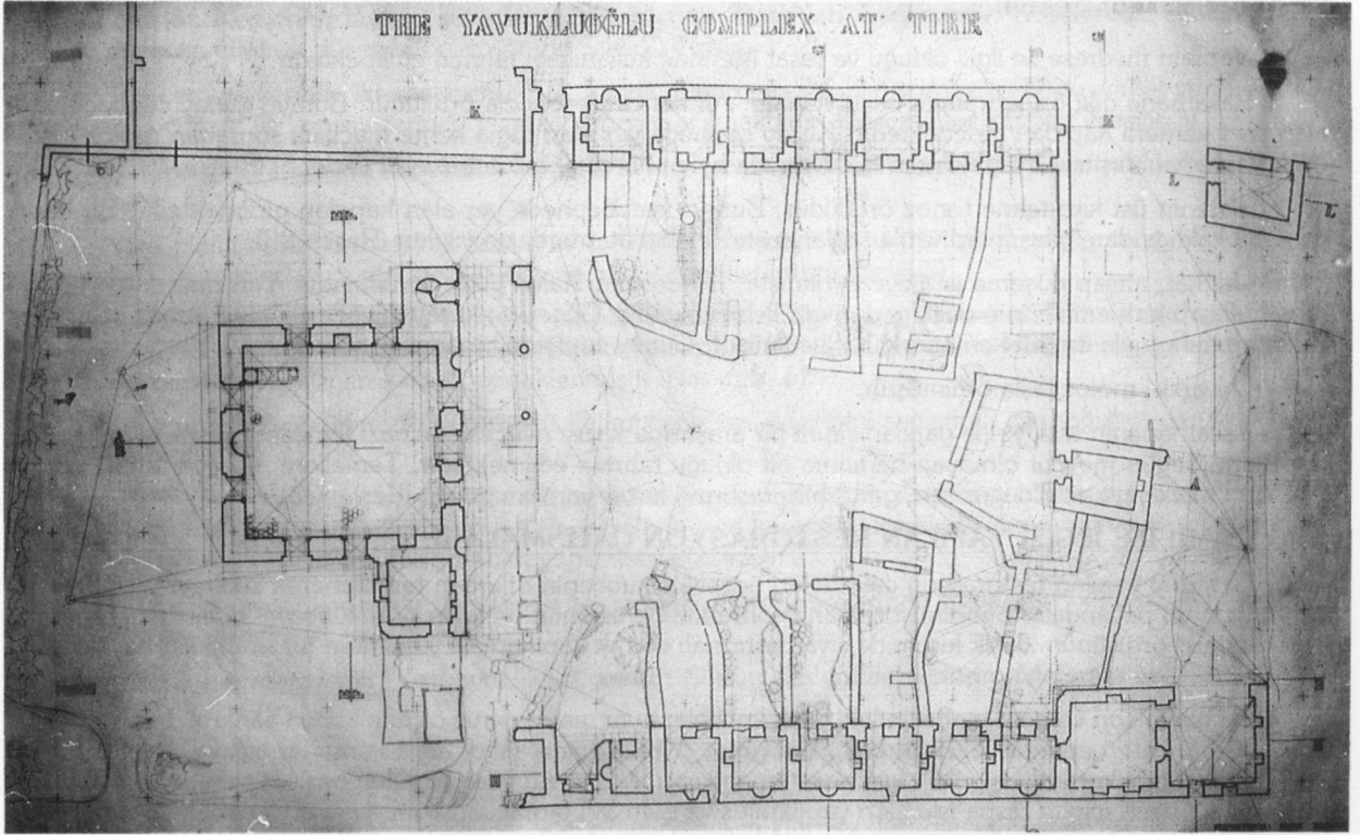
Şekil : 1. İzmir ili, Tire İlçesi'nde bulunan Yavukluoğlu (Yoğurtluoğlu) Külliyesinin genel planı. (Yakup HAZAN)
