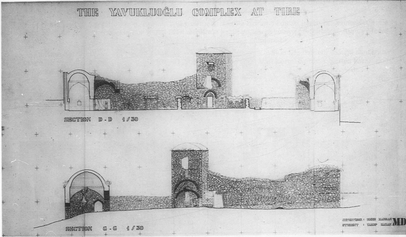
Şekil 4. Külliye dahil rasathanenin güney ve kuzey cephelerinin rölöve görüntüleri. (Yakup HAZAN)
