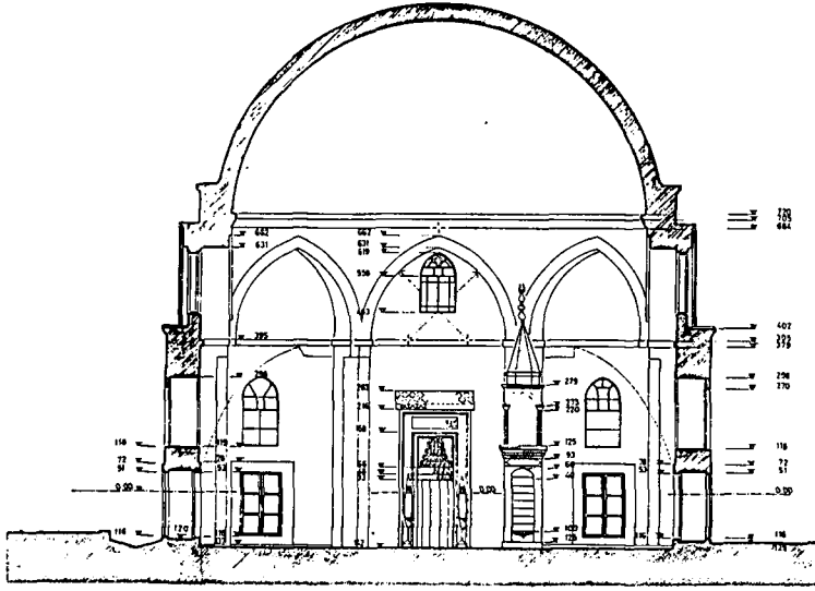
A - A Kesiti 1/50
