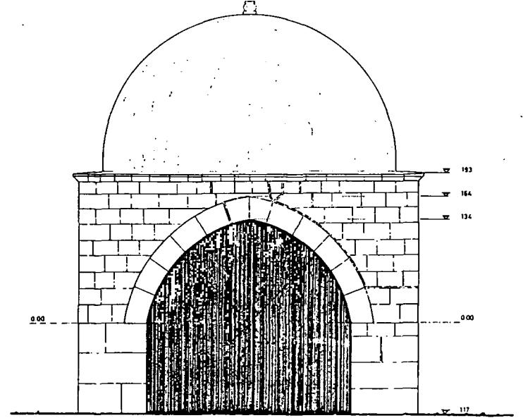
Kuzey Cephe 1/20
