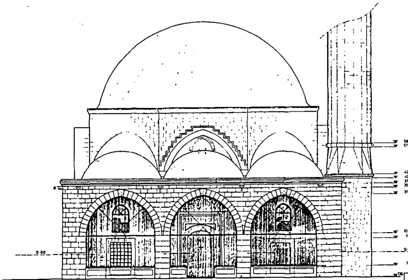
Kuzey(Giris) Cephe 1/50
