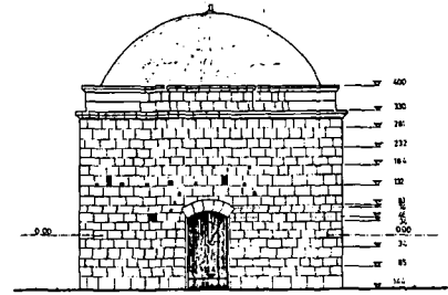
Doğu (Giriş) Cephesi 1/50
