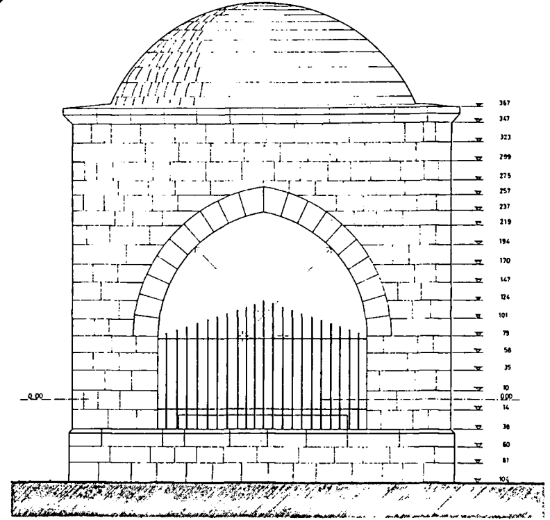
Kuzey Cephe 1/20
