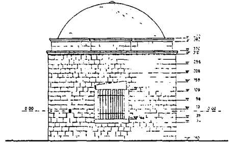
Batı Cephesi 1/50
