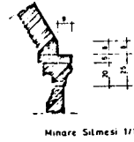
MİNARE SİLMESİ 1/10
