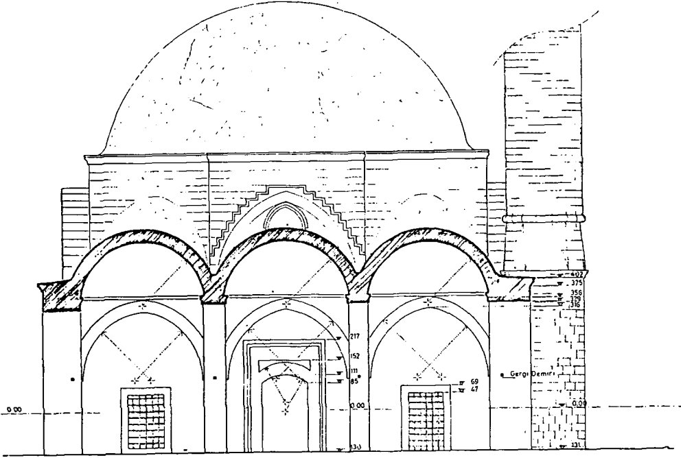
C - C Kesiti 1/50
