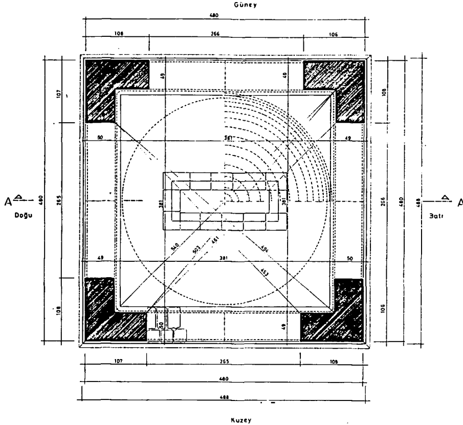
Plan 1/20
