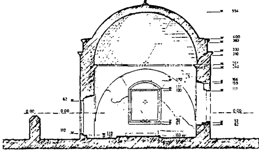
A - A Kesiti 1/50
