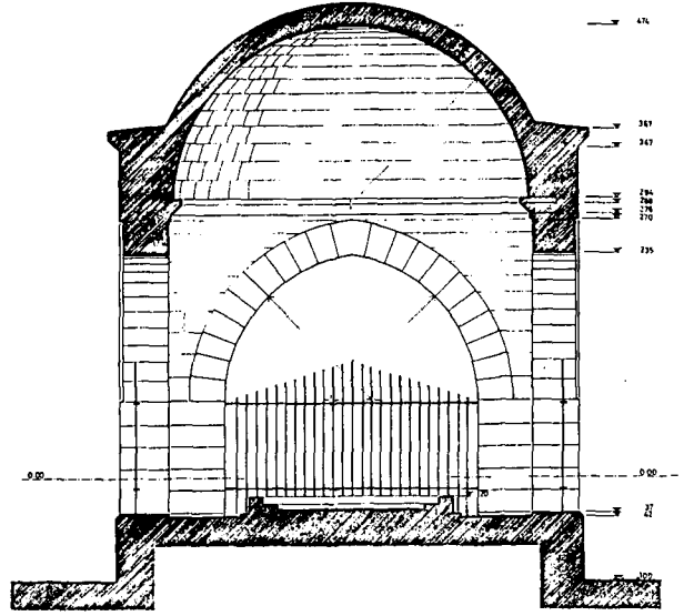
A-A Kesiti 1/20
