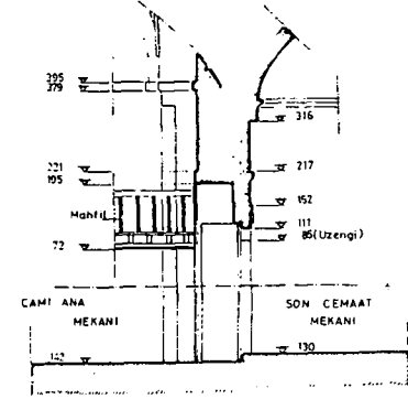
3 Detay 1/50
