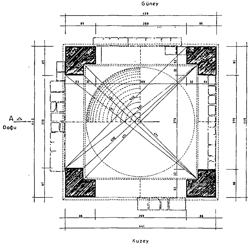
PLAN 1/20
