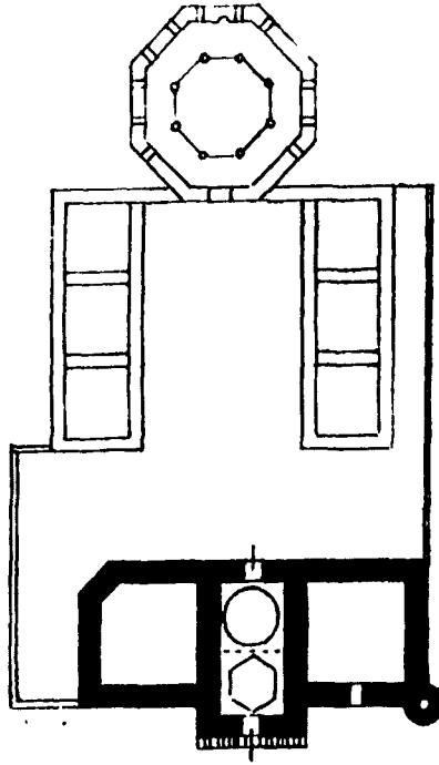
Resim : 4 — Çankırı Darüşşifasında, mevlevihane Semahanesi ve Taş Mescit itlak olunan kısım ile Darüşşifa odalarının takribi plânı. (A. Kemal)
