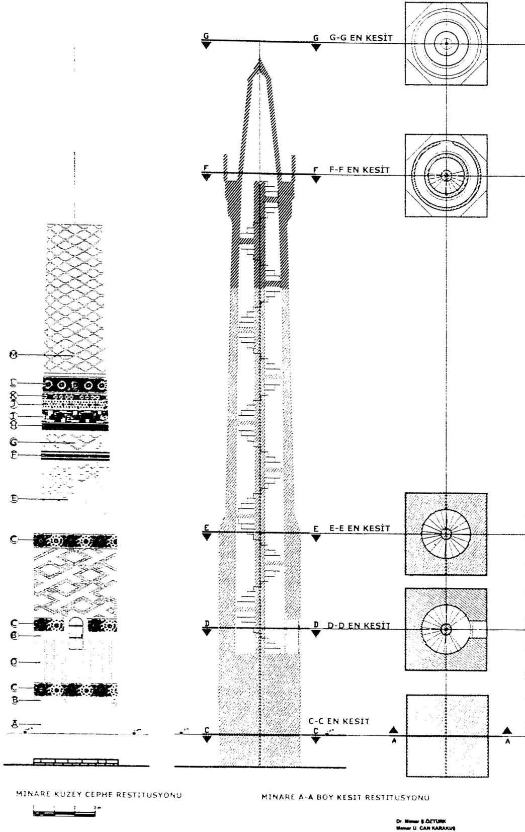
Çiz. 4 Siirt Ulu Cami Minaresi Restitüsyonu.
