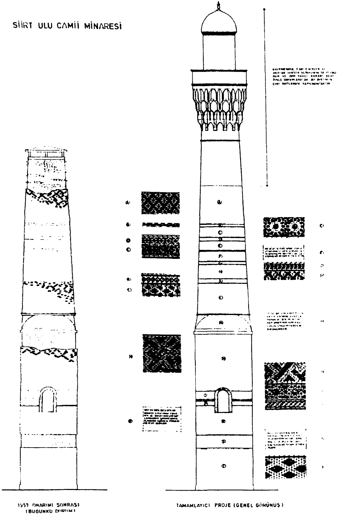
Çiz. 2 Siirt Ulu Cami Minare Rölövesi (İ. Köprülü - U.Ünal'dan).
