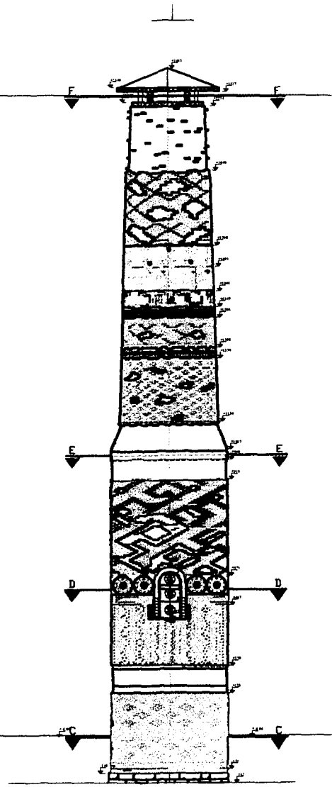
MİNARE KUZAY CEPHE RÖLÖVESİ
