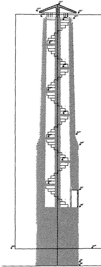
MİNARE A-A BOY KESİT RÖLÖVESİ
