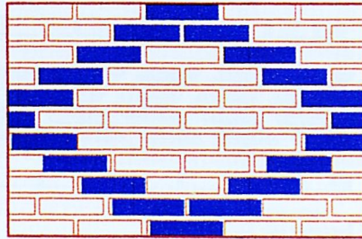
M-DETAYI
