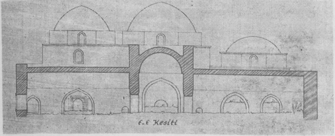
Resim : 8 — Siirt Ulu Camii rölövesi : E-E. kesiti.
