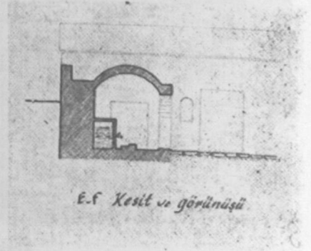
Resim : 5 — Siirt Ulu Camii rölövesi : E-F. kesit ve görünüşü.
