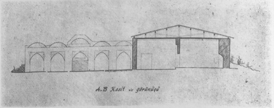
Resim : 3 — Siirt Ulu Camii rölövesi : A.B. kesit görünüşü.
