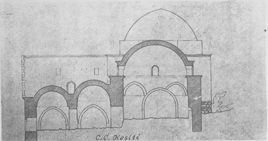
Resim : 9 — Siirt Ulu Camii rölövesi : C-C'. kesiti.
