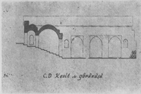
Resim : 4 — Siirt Ulu Camii rölövesi : C-D kesit ve görünüşü.
