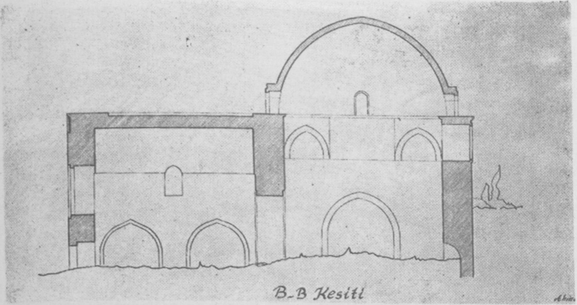
Resim : 7 — Siirt Ulu Camii rölövesi : B-B. kesiti.
