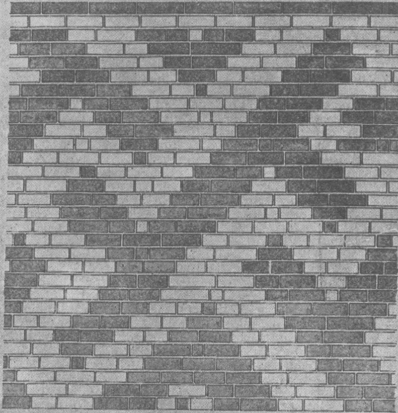
MİNARENİN KAİDEDEKİ MOTİFLERİ ÖLÇEK 1/5
