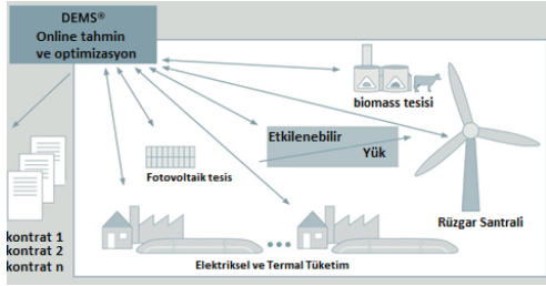
Şekil 4: Dağıtık Üretim Yönetim Sistemi (DEMS)
