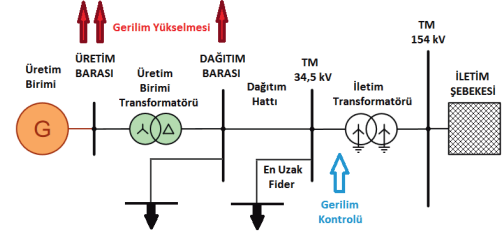
Şekil 2: Üretim entegrasyonları sonucu oluşabilecek gerilim yükselmesinin resmedilmesi
