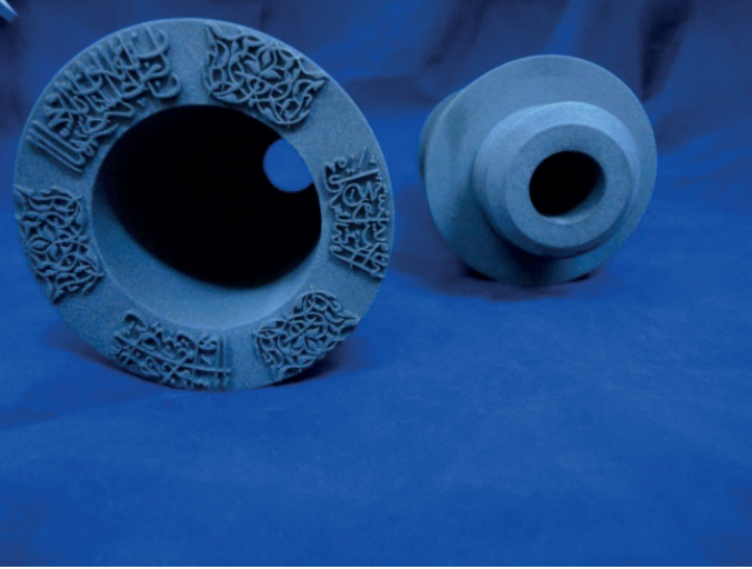
Resim 8. Laboratuvarıda ürettiğimiz iki parçalı Şahi Topu modeli ve tam detaylı alın yazısı.
