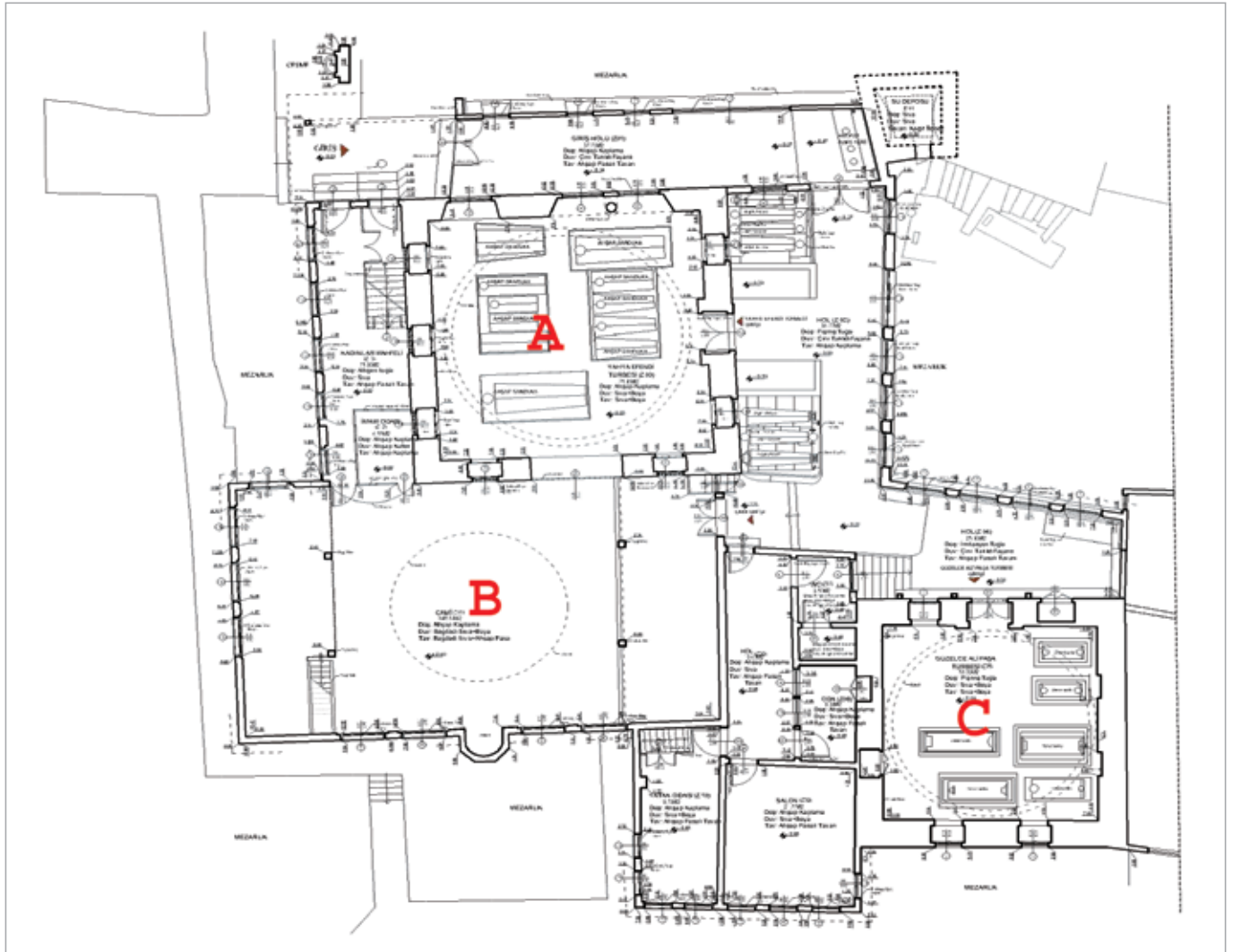
Plan 2-Yahya Efendi Türbesi, Güzelce Ali Paşa Türbesi ve Camiye ait Rölöve planı (Pekerler İnş. Tic. San. Ltd. Şti tarafından hazırlanmıştır.)
