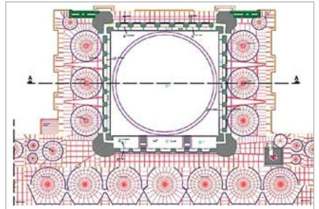
Çizim,5-Kot planları
