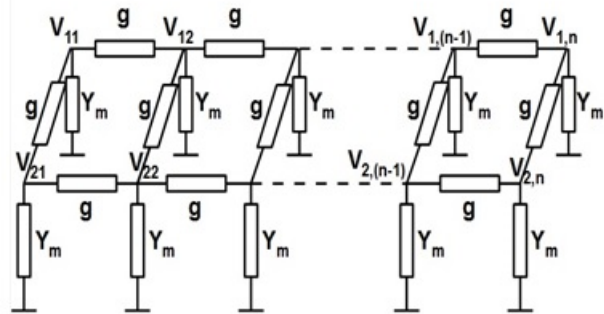
Şekil 1. İki boyutlu nöron ağının elektriksel modeli
