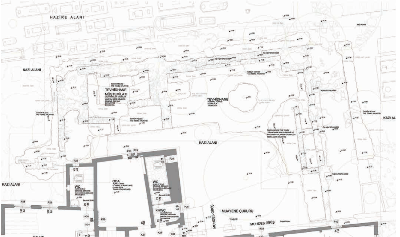
Şekil 5. Kademî Şerîf Tekkesi kazı sonrası röleve (Çizen:ATA Proje)
