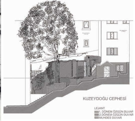
Şekil 16. Kuzeydoğu cephesi (Natura Restorasyon-Mimarlık)
