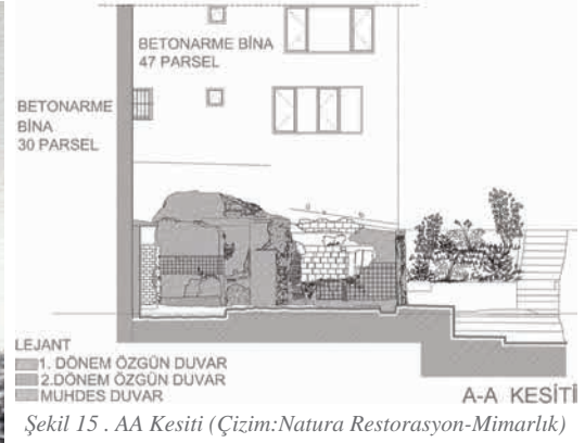
Şekil 15 . AA Kesiti (Çizim:Natura Restorasyon-Mimarlık)
