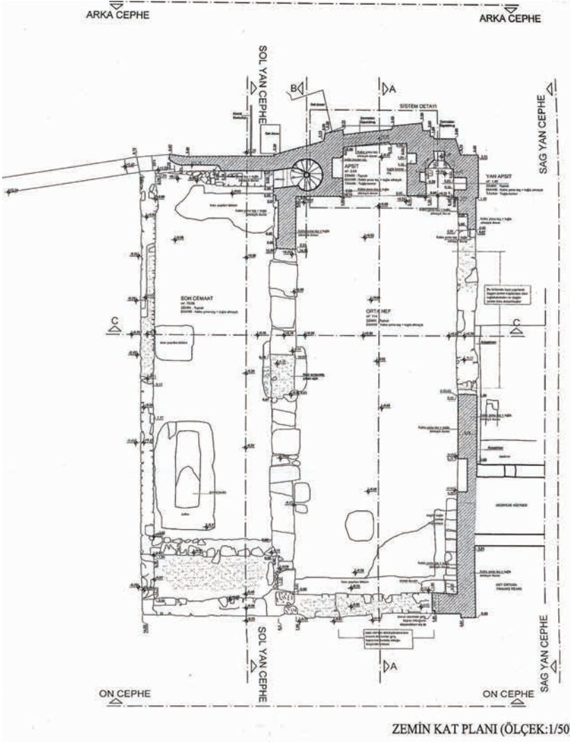
Şekil 20. İsakapı Mescidi zemin kat planı (Çizim:Taksim Yapı).
