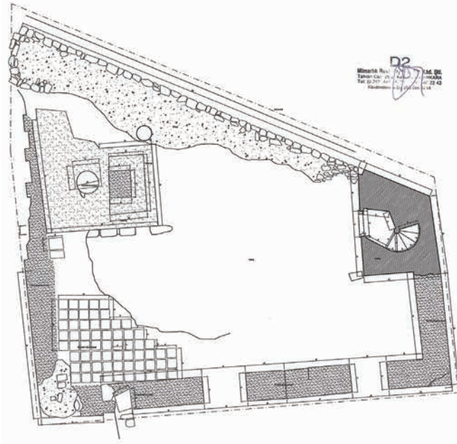
Şekil 4 .Hacı İlyas Mescidine ait rölöve (Çizim:D2 Mimarlık)
