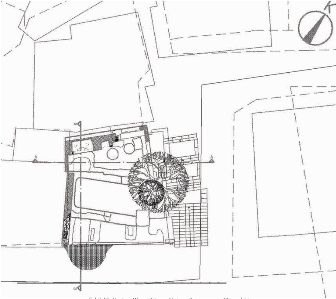
Şekil 12. Vaziyet Planı (Çizen: Natura Restorasyon-Mimarlık)
