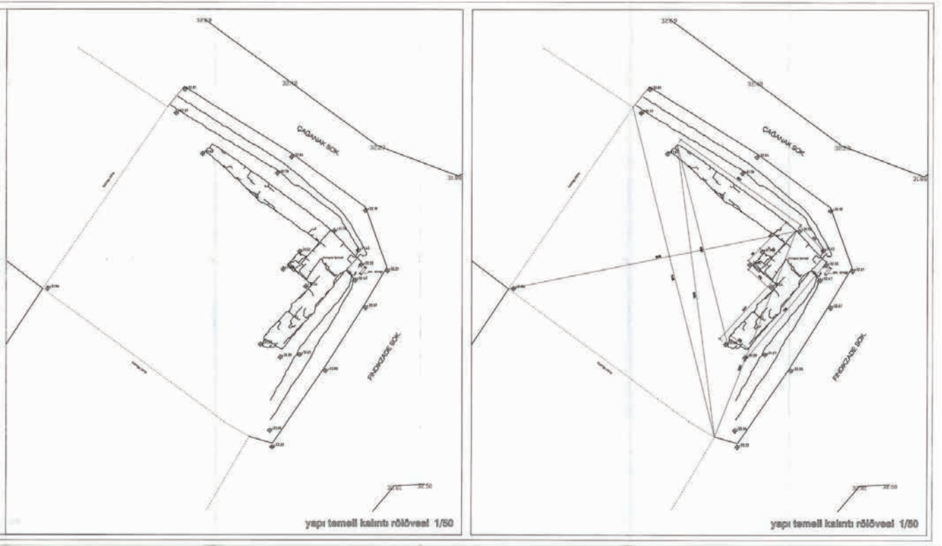
Şekil 11 .Seydi Bey Mescidine ait temel kalıntı rölövesi (Çizen: Mehmet Raif Doğan Mimarlık)
