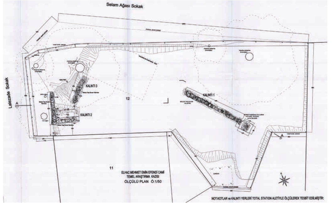
Şekil 8 . Arkeolojik kazı rölövesi (Çizim: MC Mimarlık)
