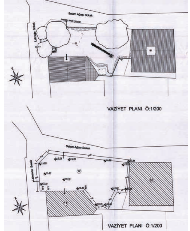
Şekil 7. Simkeş Mescidi Vaziyet Planı (çizim: MC Mimarlık)
