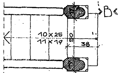
Çizim 4: Alaca Camii minber detayı.
