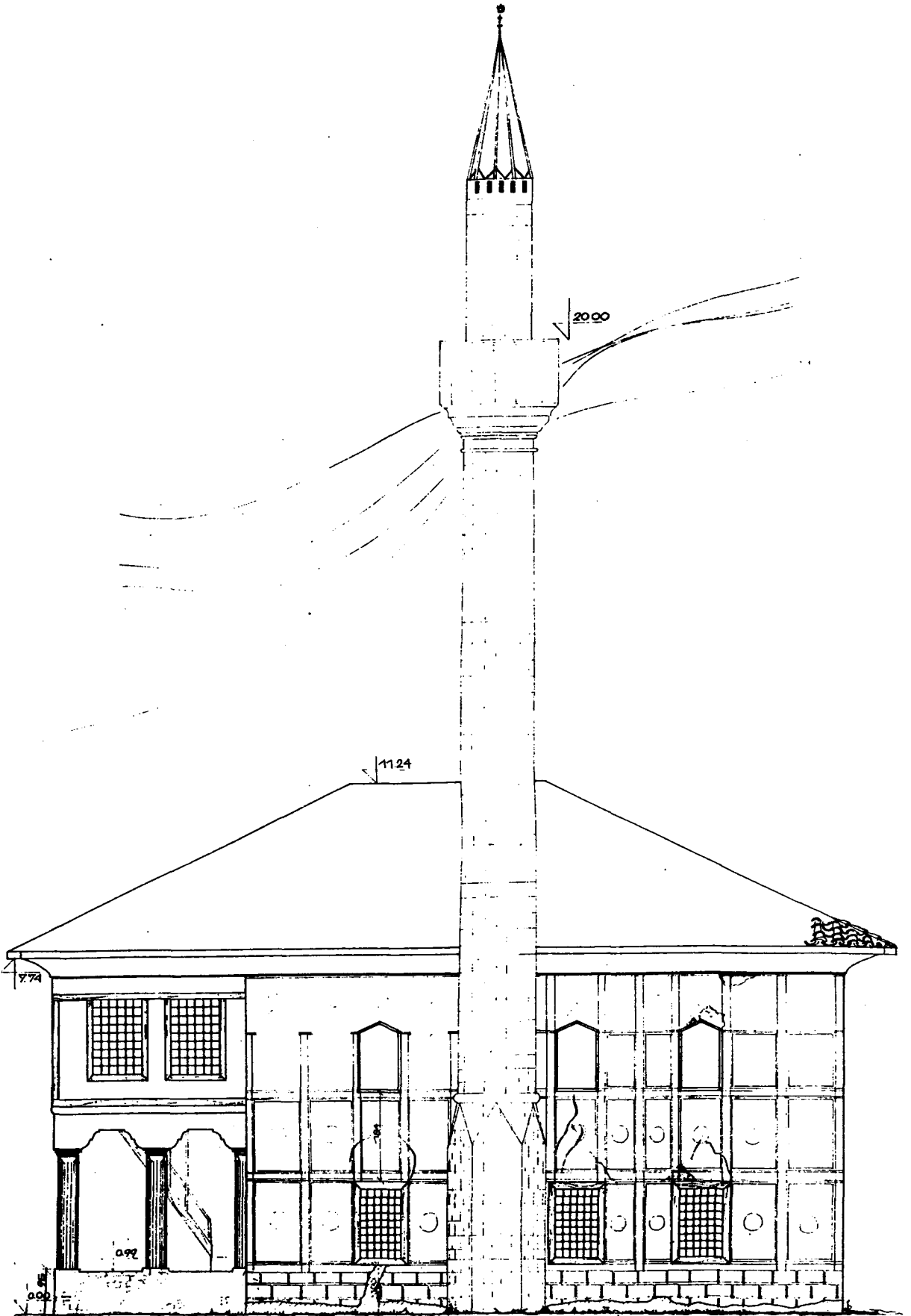
Çizim 6: Alaca Camii batı cephesi.
