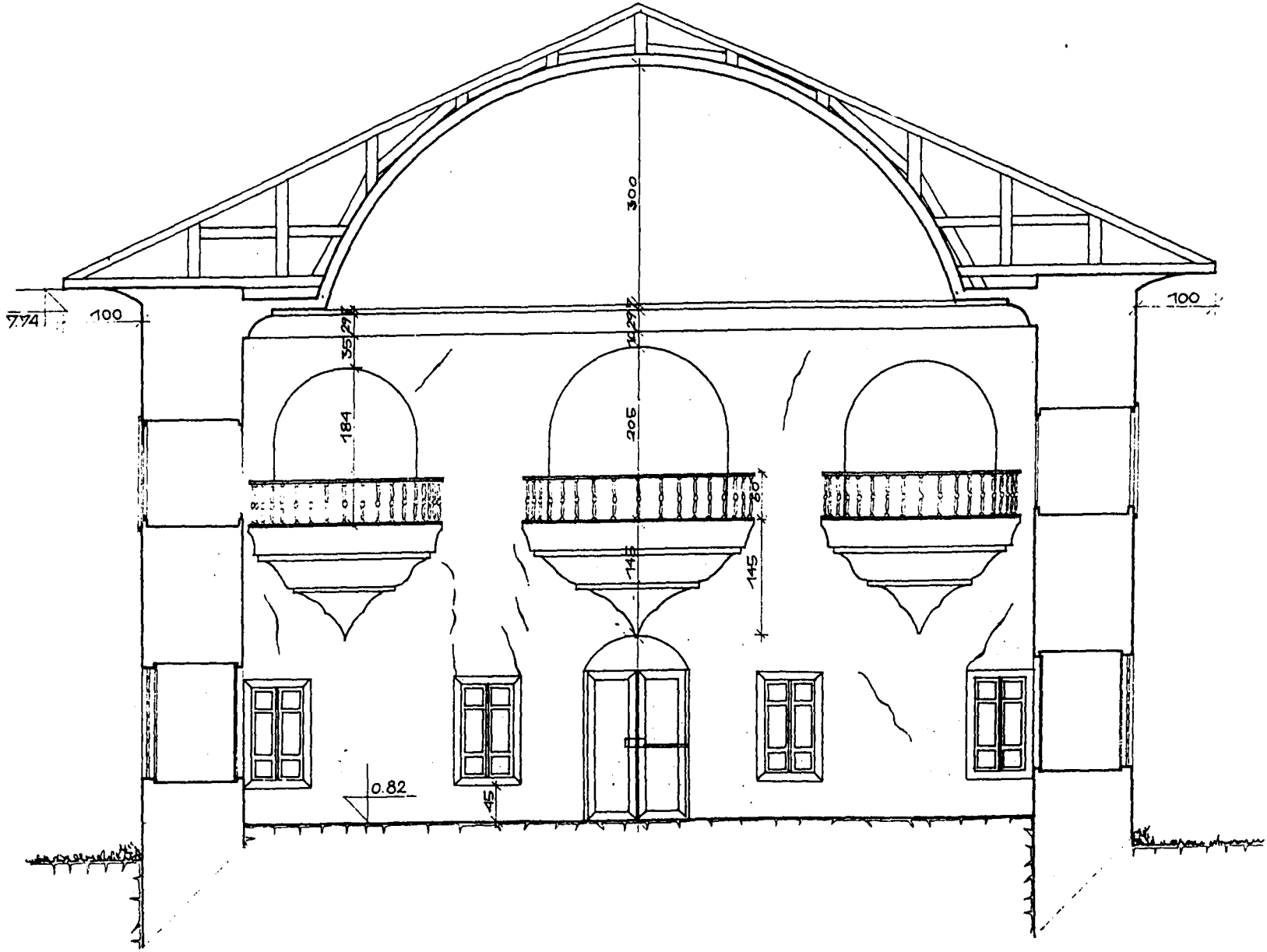
Çizim 3: Alaca Camii'nin kuzey cephesini gösterir kesit.
