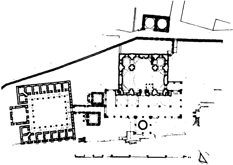
9- Istanbul, Üsküdar, Mihriman Sultan Külliyesi planı (Kuran'dan)
