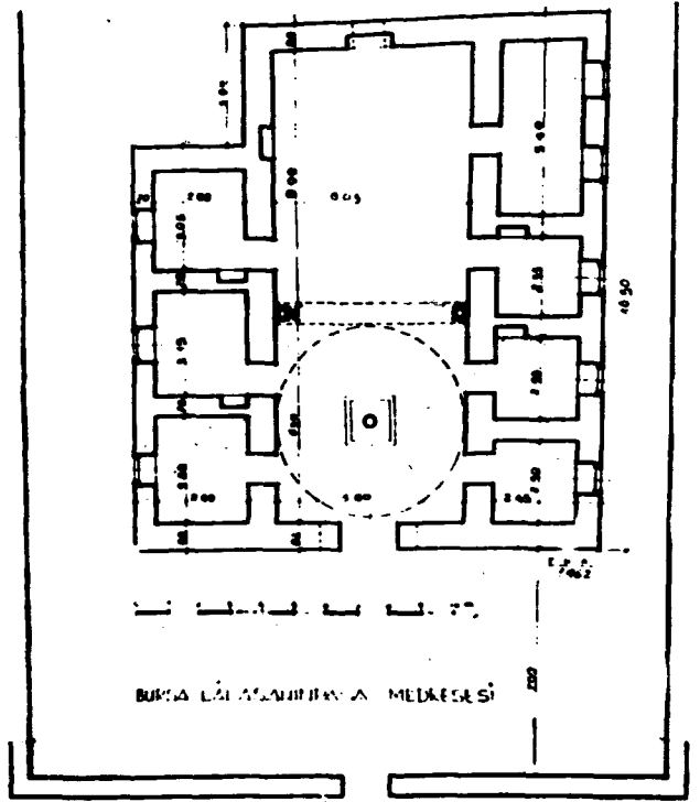
2- Bursa, Lala Şahin Paşa Medresesi planı (E.H.A. dan)
