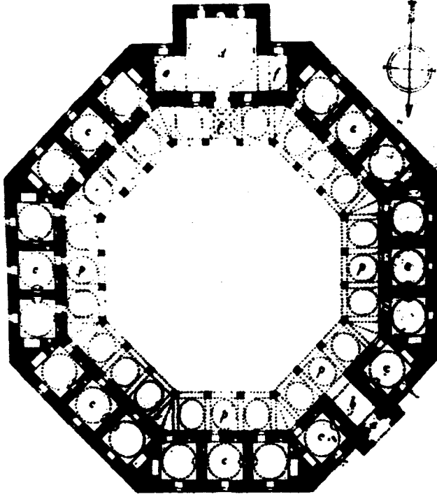
5- Amasya, Kapiağası Medresesi planı
